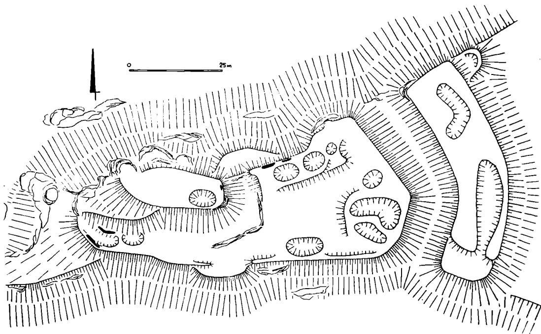
Obr. 10. Jevišovice-Starý hrad, terénní náčrt zříceniny.
