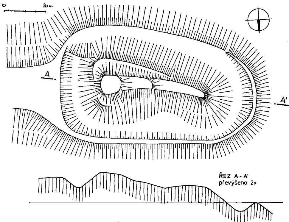
Obr. 4. Drnholec, terénní náčrt hrádku.
