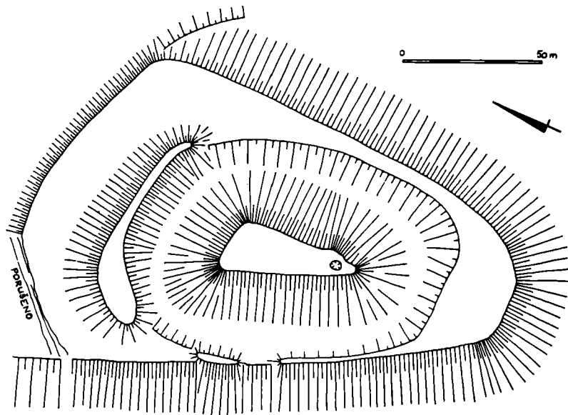
Obr. 3. Haslach-Dernberg, terénní náčrt hrádku.
