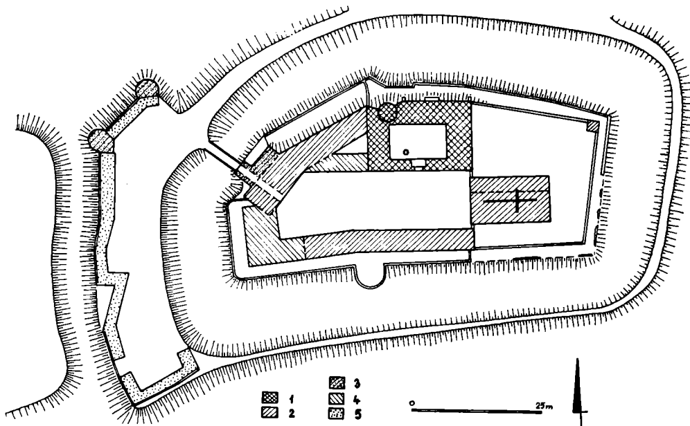
Obr. 8. Mallberg, vývojové schéma hradu. 1 — budova komendy, 2 — v jádru gotické objekty, 3 — objekty z 15. sto- letí, 4 — renesanční a barok- ní budovy, 5 — pozdější.
