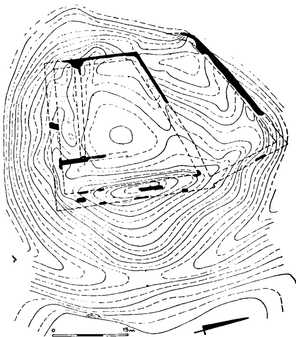
Obr. 9. Šenkenberk, půdorysné a výškoplné zaměření hradu.
