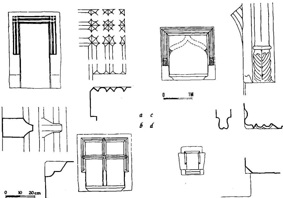
Obr. 4. Zaječice, o. Chrudim, obytné stavení, čp. 1 — portál (a), okno v přízemí (b) a v patře (c), na východním a okénko (d) na jižním průčelí obytného stavení, čp. 1. Měřítko všech celkových nárysů i všech podrobností jsou shodná.
