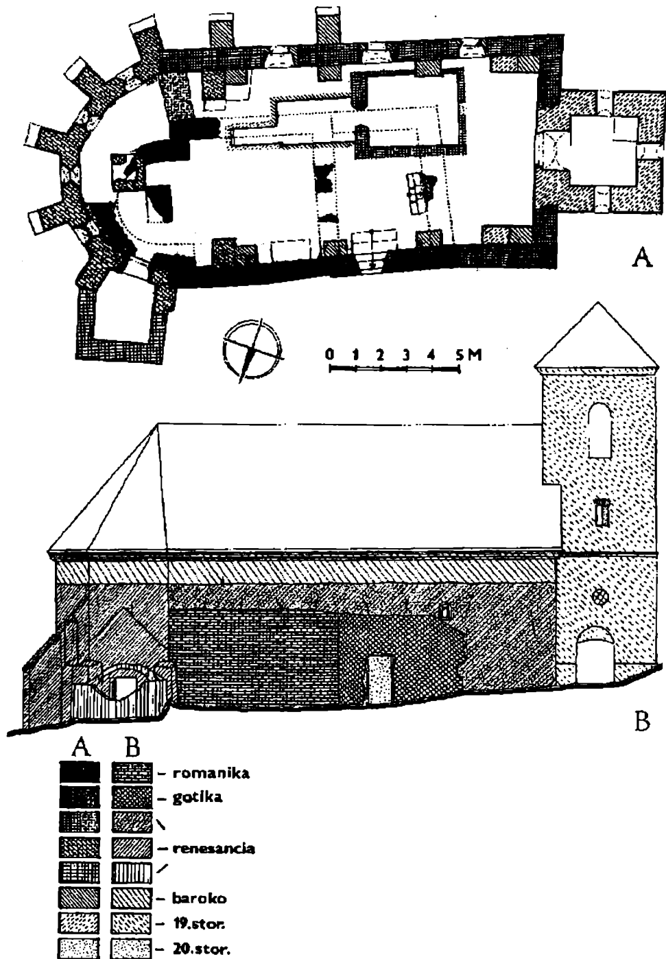
Obr. 2. D. Leľovce, r. k. kostol – pôdorys a severná fasáda so slohovou analýzou.
