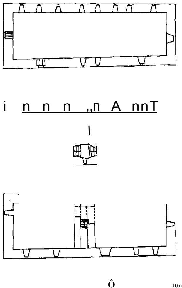
Obr. 4, Volyní, půdorysy tvrže. Zdola přízemí, 1. a 2. patro.
