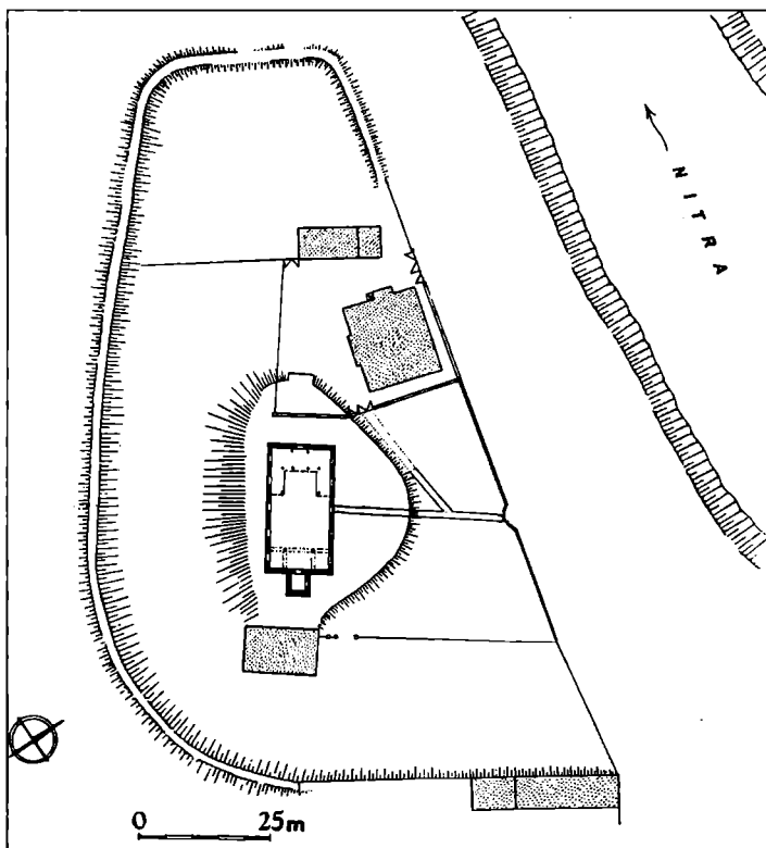
Obr. 18. Nitrianska Streda – pôdorys zvyškov hradu podľa zamerania PÚ Topoľčany v r. 1994. Kresba M. Bóna.
