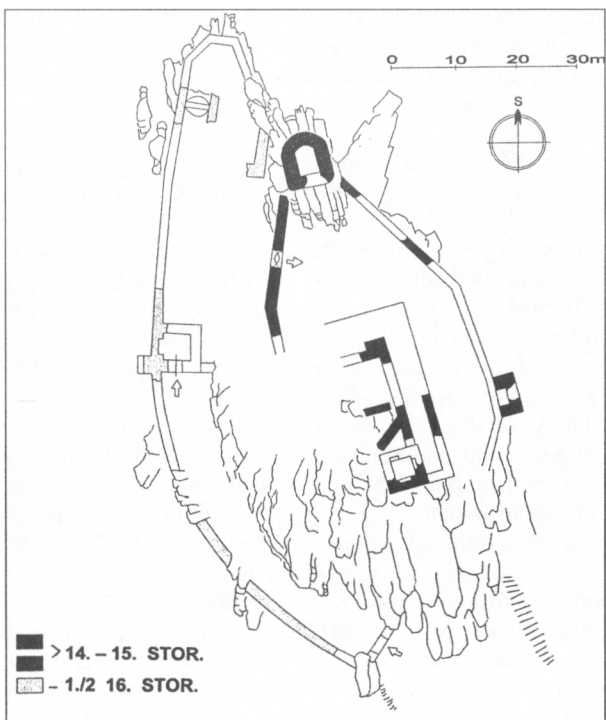
Obr. 19. Hrad Sívý Kameň – pôdorys so stavebnou etapizáciou podľa D. Menclovej z r. 1956.
