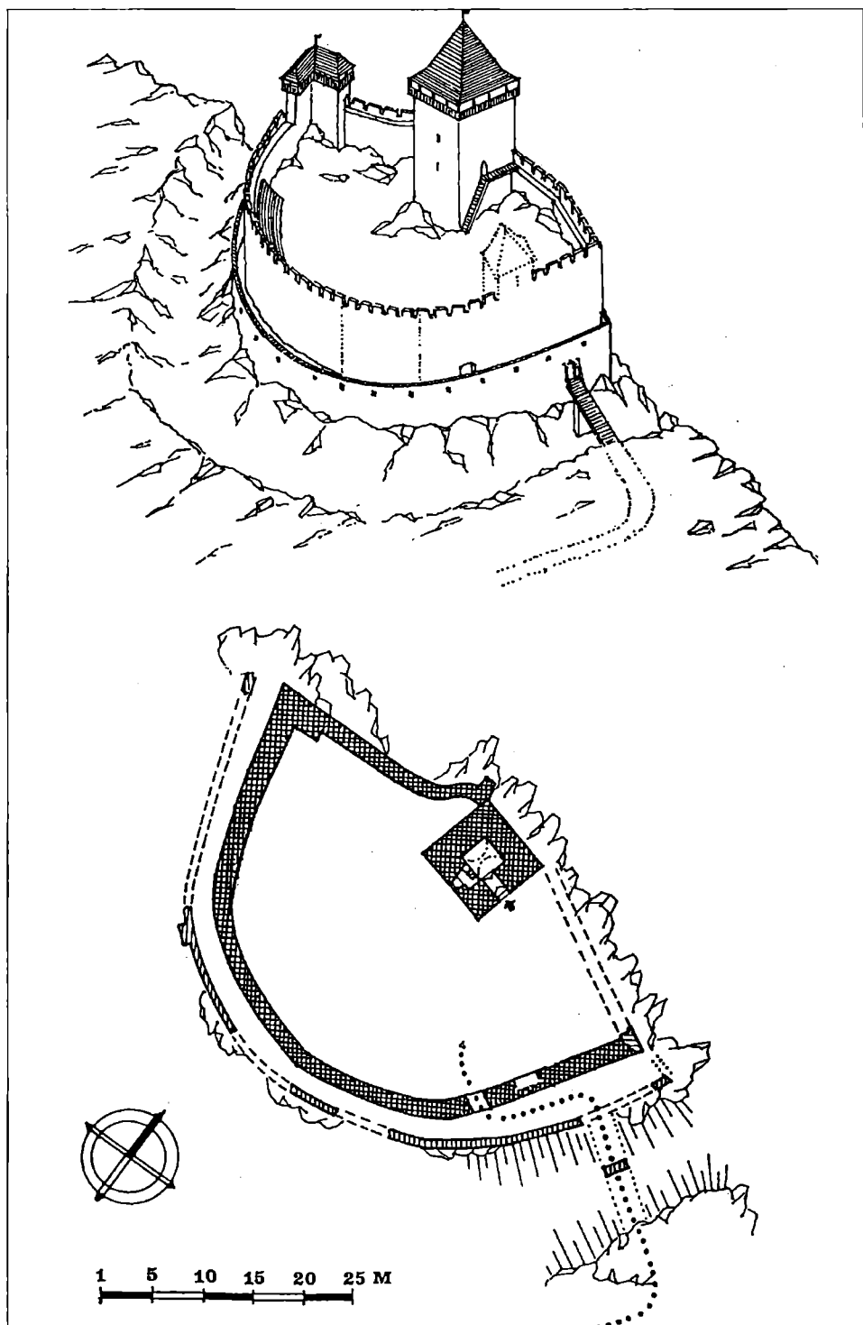
Obr. 10. Hrad Topoľčany – perspektívna a pôdorysná rekonštrukcia hradu okolo pol. 14. stor. Kresba: M. Bóna.
