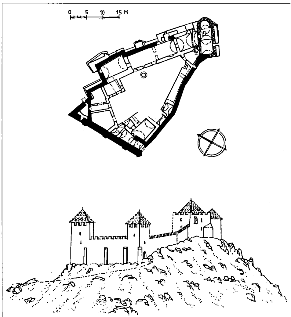
Obr. 8. Hrad Uhrovec – pôdorys hradného jadra s vyznačením murív z 2. pol. 13. stor. podľa M. Bónu–P. Horanského 1999 a rekonštruovaný juhozápadný pohľad na konci 13. stor. Kresba: M. Bóna.
