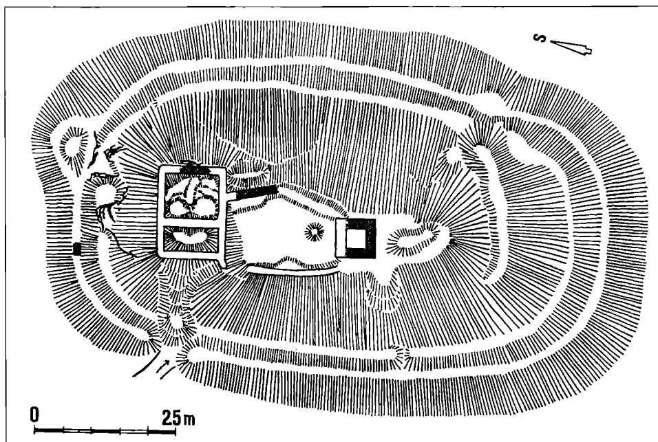
Obr. 17. Čierny hrad – pôdorysný náčrt podľa D. Menclovej z r. 1957.
