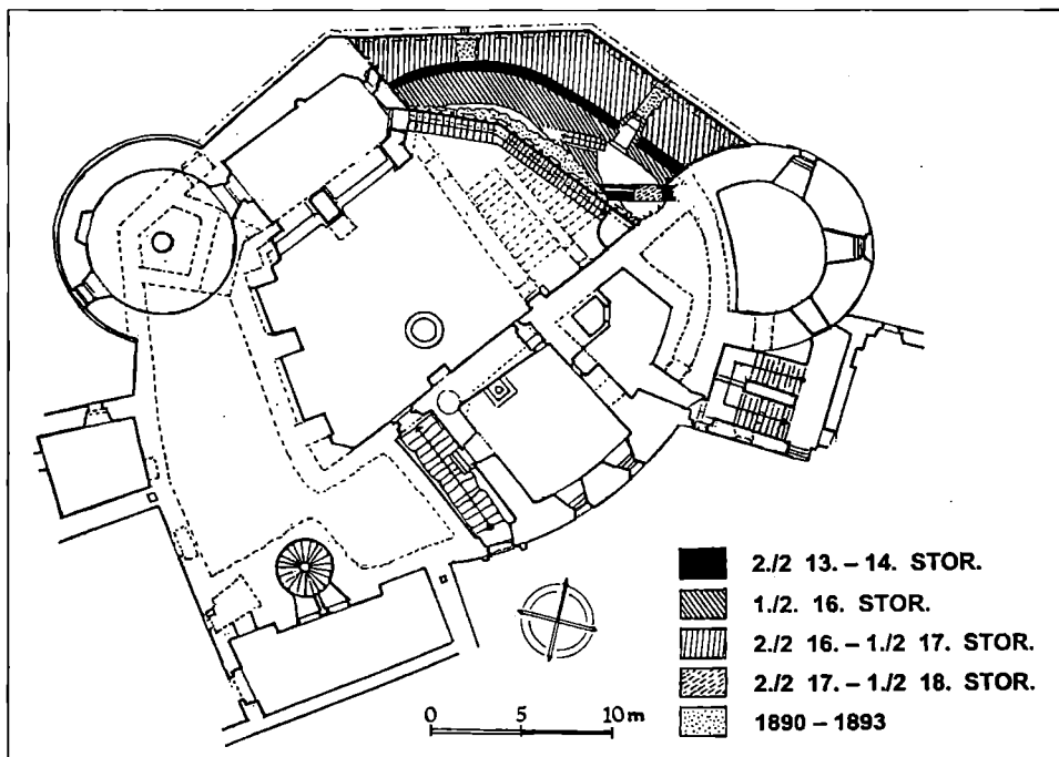
Obr. 16. Hrad Bojnice – pôdorys hradného jadra s vyznačením skúmanej plochy podľa M. Remišovej–K. Malečkovej–M. Bónu 1997.
