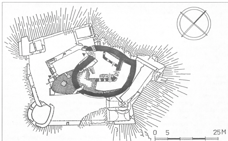
Obr. 12. Hrad Hrušov – pôdorys jadra a 1. predhradia s vyznačením murív z 13. (čierne) a 14. stor. (krížkované). Kresba: M. Bóna.
