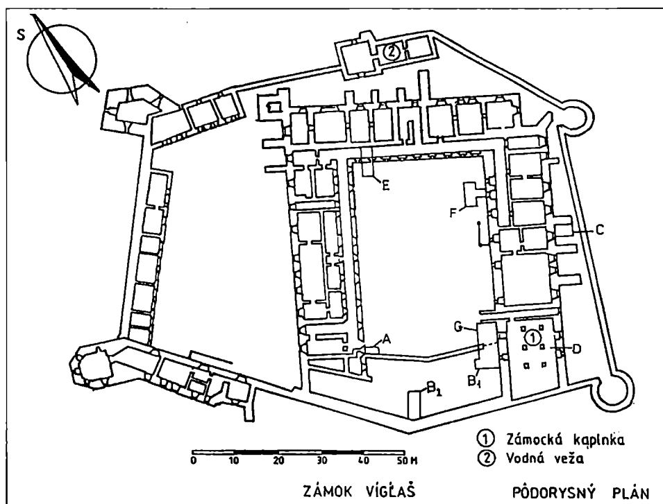
Obr. 4. Víglaš – zámok, pôdorysný plán.
