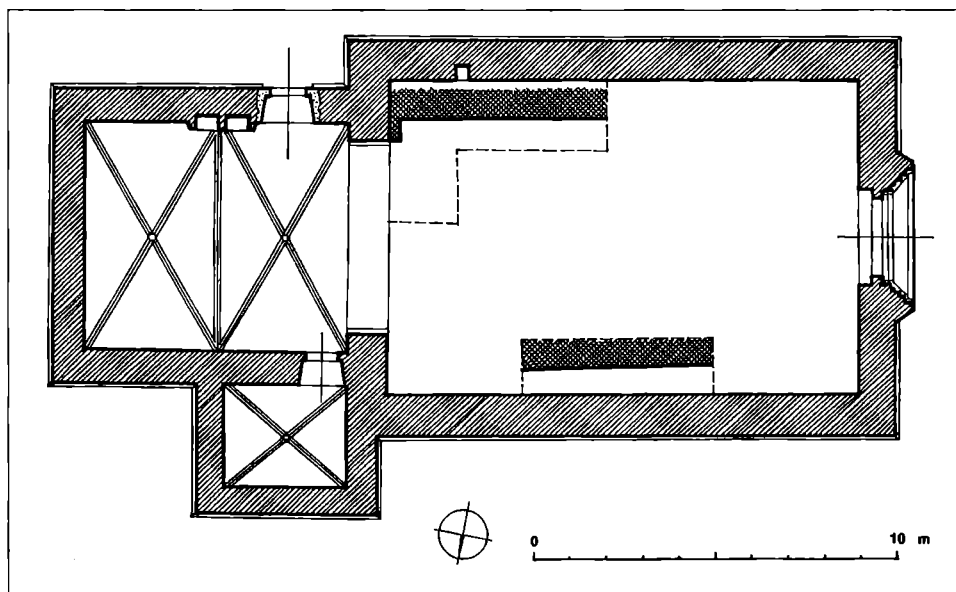
Obr. 14. Tečovice, kostel sv. Jakuba Většího – půdorys stávajícího zdiva kostela (šrafovaně) s vyznačením zdiva, odhaleného archeologickým výzkumem (křížem šrafovaně) (kresba: R. Vrla 2001).
