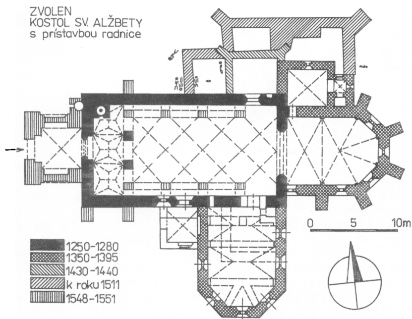
Obr. 5. Pôdorys Farského kostola sv. Alžbety a odkrytej prístavby historickej radnice. Zameral: M. Bábik, kreslil: H. Michelčík.
