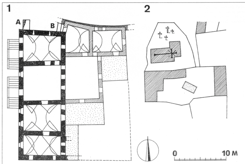
Obr. 4. Tlumačov: 1 – Panský dům, půdorys v úrovni přízemí s orientačním vyznačením předpokládaného stáří zděných konstrukcí; křížem šrafováno – starší ohradní zeď hřbitova, zrněně – konec 15. století (?), šrafovaně – 2. polovina 16. století, tečkovaně – mladší přístavby; přerušovanou čarou vyznačen předpokládaný rozsah tvrze do počátku 17. století; A, B – poloha archeologických sond; 2 – výřez z indikační skici (1830), nahoře kostel sv. Martina, dole Panský dům.
