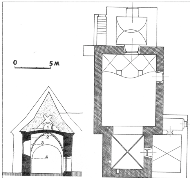
Obr. 5. Tlumačov – kostel sv. Martina; vlevo – svislý řez vedený příčnou osou presbytáře; 1 – průchod ve východním štítu lodi (přerušovanou čarou zaznačena poloha kapsy po závoře, nad průchodem vyznačen obrys staré střešní konstrukce, tečkovaná plocha exteriérových omítek v prostoru krovu); 2 – horní úroveň záklenku hrotitého okna; 3 – vrchol starší klenby (dle situace na jižní stěně presbytáře); 4 – úroveň parapetu staršího okna; vpravo – půdorys s vyznačením středověkých konstrukcí (stáří opěrného pilíře u jihozápadního nároží lodi je v současné době nezjistitelné).
