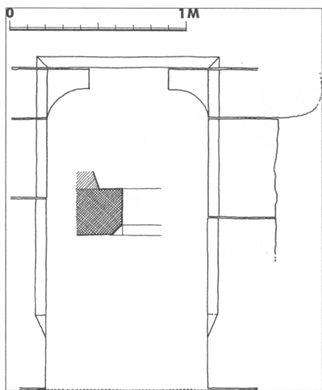
Obr. 11. Břežnice – kostel sv. Bartoloměje; zaměření gotického ostění vstupu do sakristie – pohled od jihu a profil.
