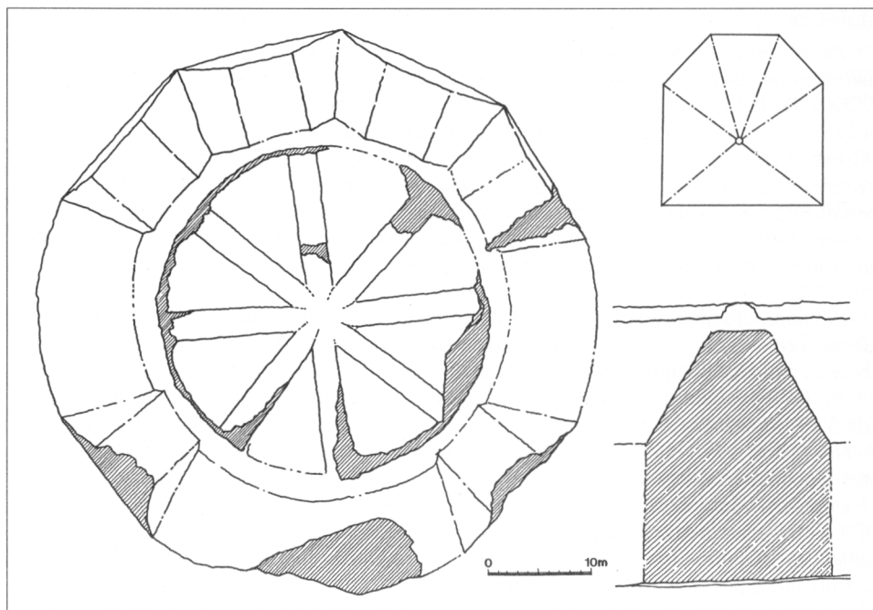
Obr. 13. Slušovice – zaměření klenebního svorníku, vpravo dole profil žebra, vpravo nahoře pokus o rekonstrukci klenebního obrazce a půdorysu presbytáře.
