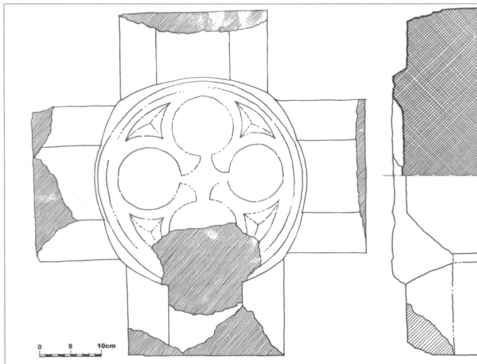
Obr. 15. Mysločovice – zaměření klenebního svorníku, vpravo svislý řez (nahore) a boční pohled (dole).
