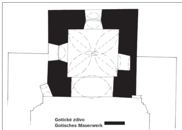
Obr. 1. Stráž pod Ralskem, kostel sv. Zikmunda. Horizontální řez prvním patrem věže s vyznačeným gotickým zdívem. Zaměření T. Nejezchlebová.
