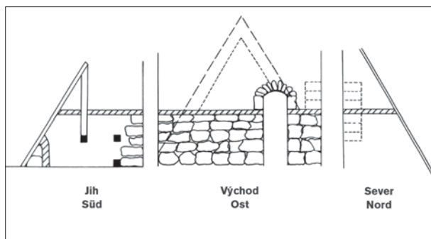
Obr. 2. Stráž pod Ralskem, kostel sv. Zikmunda. Skica situace gotických reliktvé ve třetím patře věže při pohledu z podkrovní lodě (1:50). Zaměření T. Nejezchlebová, I. Peřina.
