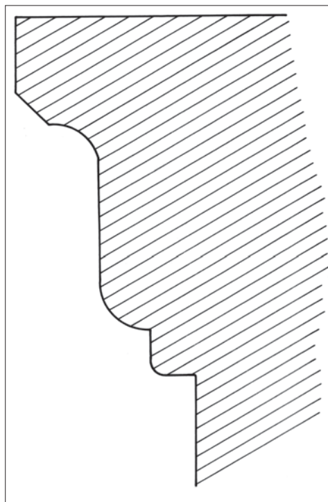
Obr. 3. Stráž pod Ralskem, kostel sv. Zikmunda. Profil gotické římsy ve třetím poschodí věže (1:2). Zaměření T. Nejezchlebová.
