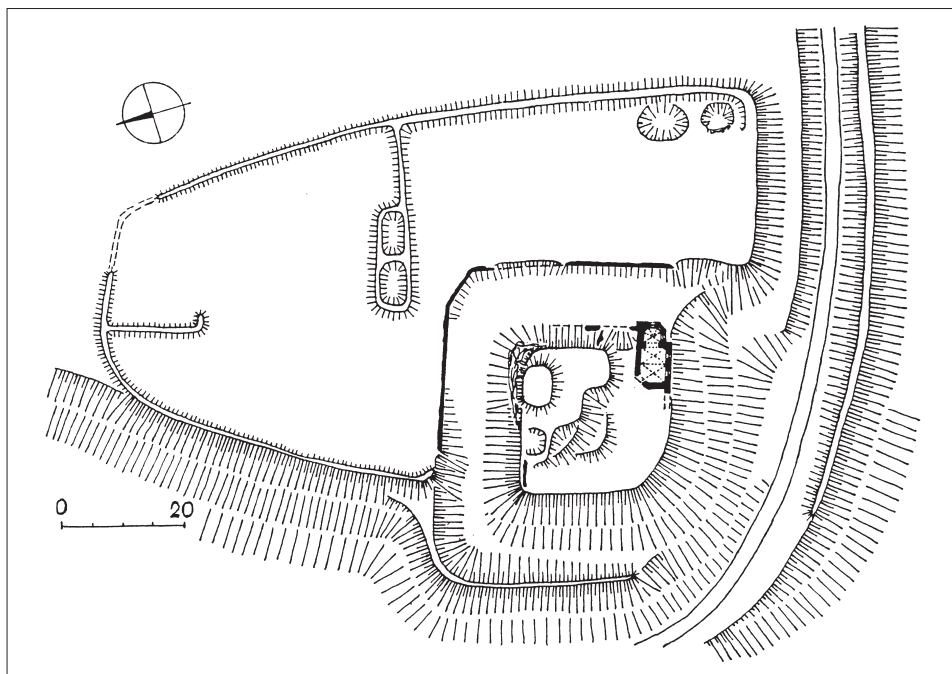
Obr. 9. Gaber, náčrt půdorysu zbytků tvrze a dvora (k. ú. Luden).
