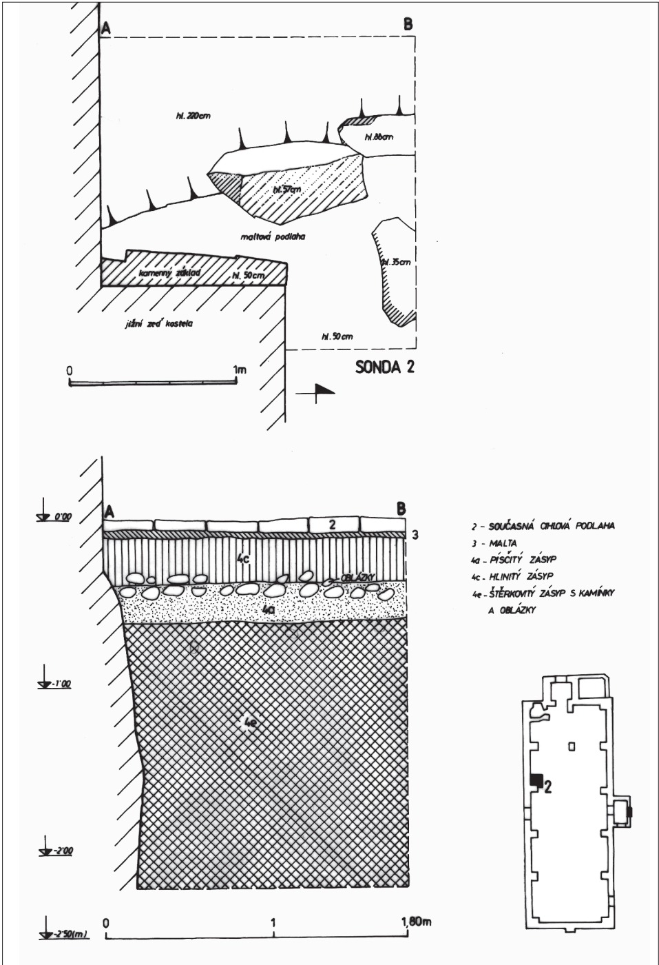
Obr. 8. Kostel sv. Markéty ve Strakonících. Půdorys a profil sondy S-2/95. Kresba J. Michálek a B. Nechvátal. Abb. 8. St. Margarethenkirche. Grundriss und Profil von Sonde S-2/95. Zeichnung J. Michálek und B. Nechvátal.
