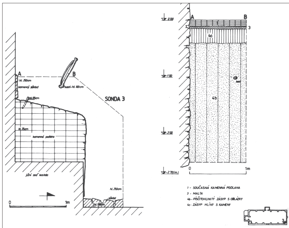
Obr. 9. Kostel sv. Markěty ve Strakonících. Půdorys a profil sondy S-3/95. Kresba J. Michálek a B. Nechvátal. Abb. 9. St. Margarethenkirche. Grundriss und Profil von Sonde S-3/95. Zeichnung J. Michálek und B. Nechvátal.
