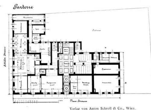
8 – Karl Grünanger, soutěžní architektonický projekt na Německý spolkový dům, 1901. Nárys fasády orientované do Komenského ulice, půdorysy 1. a 2. patra, nárys průčelí do Hlavní třídy, půdorys přízemí. Der Architekt VII, 1901
