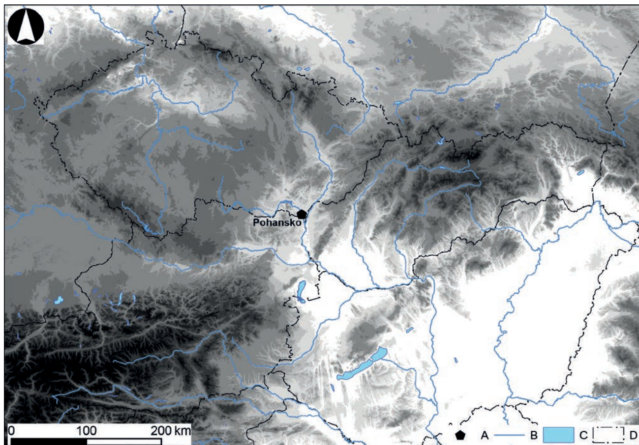
Obr. 1. Břeclav – Pohansko. Mapa s lokalizací hradiška na podkladu digitálního výškopisu střední Evropy. Legenda: A – Pohansko u Břeclavi, B – vodní toky, C – vodní plochy, D – státní hranice.
