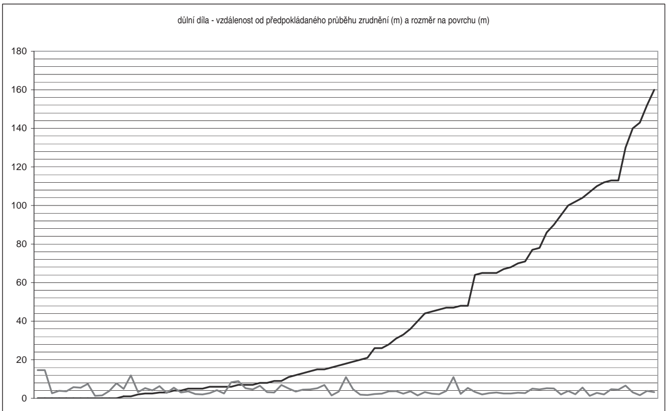
Graf. 8. Přímá povrchová vzdálenost jednotlivých jam od předpokládaného průběhu zrudnění v severní části starohorského zlomu (modrá) a rozměry jam na povrchu (růžová).
