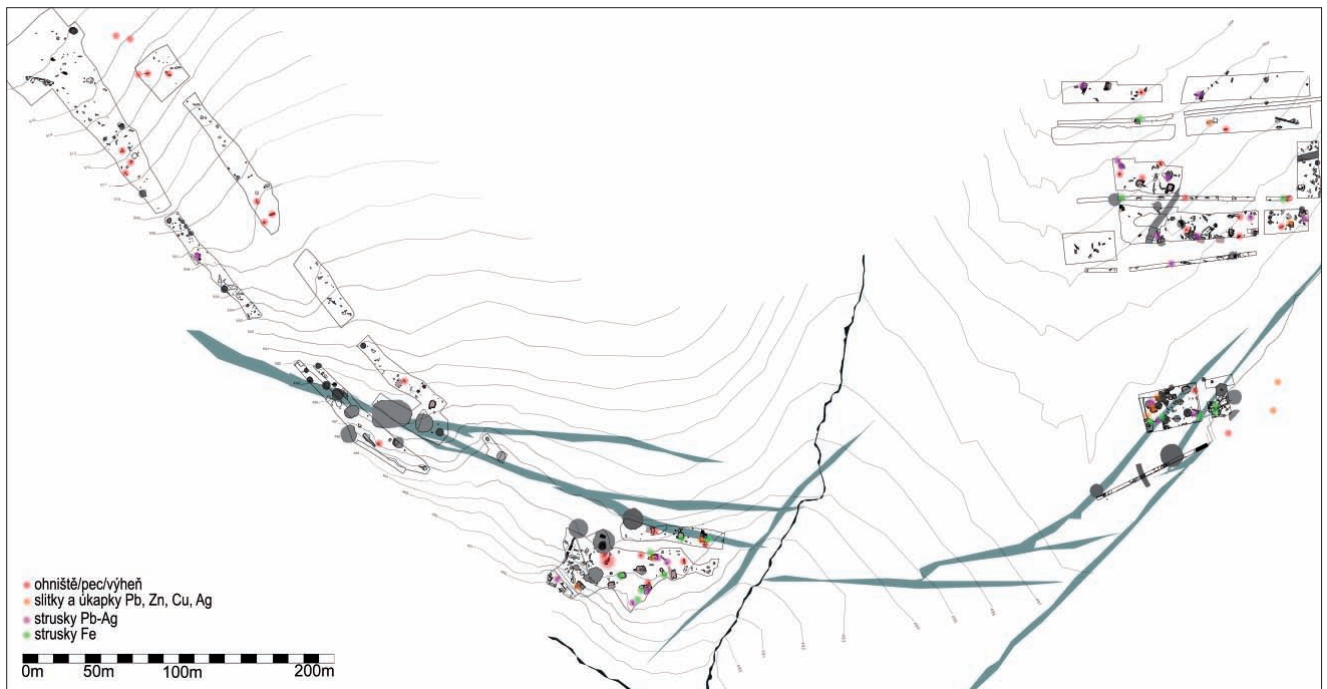
Obr. 232. Jihlava – Staré Hory, celkový plán lokalit I a III s vynesním pravděpodobných pozůstatků pecí, výhni a dalších zařízení a s vynesním rozložení archeometalurgických nálezů.
