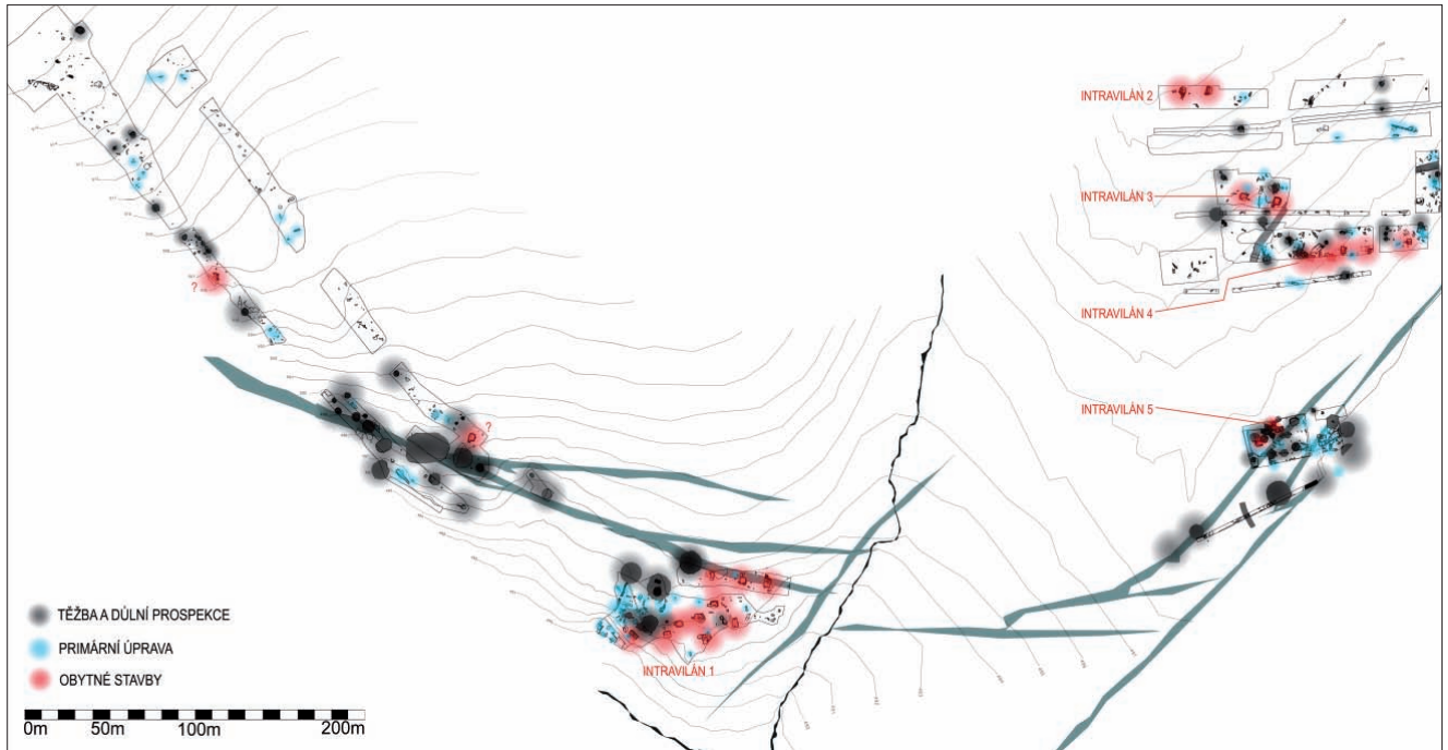
Obr. 231. Jihlava – Staré Hory, celkový plán archeologicky zkoumaných lokalit I a III s vynesním modelovaných pracovních (důlních a úpravnických) a smíšených obytných areálů. Areály těžby jsou modelovány podle hypoteticky předpokládaného maximálního rozsahu někdejších obvalů kolem jam s připočteným minimálním pracovním prostorem okolo nich. Areály primární úpravy jsou modelovány rovněž podle předpokládaného manipulačního prostoru okolo ohnišť, pecí, mlýnů, třídíren či prádel v rozsahu metrů. Obytné areály a areály hypoteticky předpokládaného hospodářství okolo zaniklých staveb jsou modelovány v rozsahu 10–15 m.
