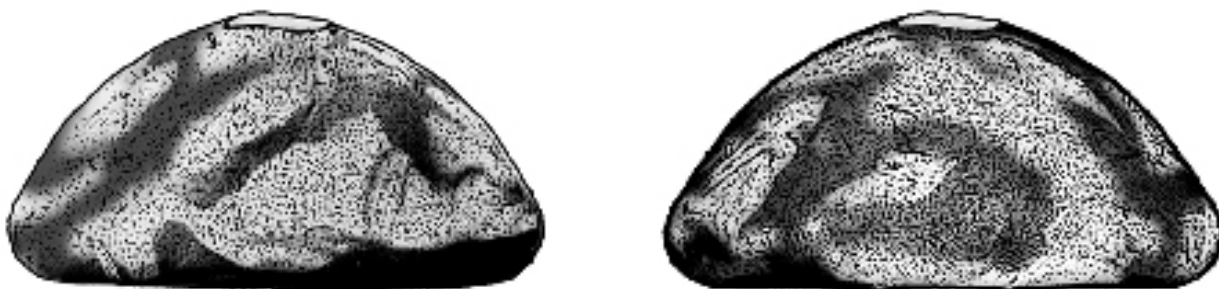
Obr. 6. Možná podoba leštěných a naleptaných hlavic vyrobených z nehomogenního železa (lokálně s vyššími obsahy fosforu). Kresba J. Hošek. Abb. 6. Mögliche Gestalt von polierten und geätzten, aus inhomogenem Eisen hergestellten Knäufen (stellenweise mit höherem Phosphorgehalt). Zeichnung J. Hošek
