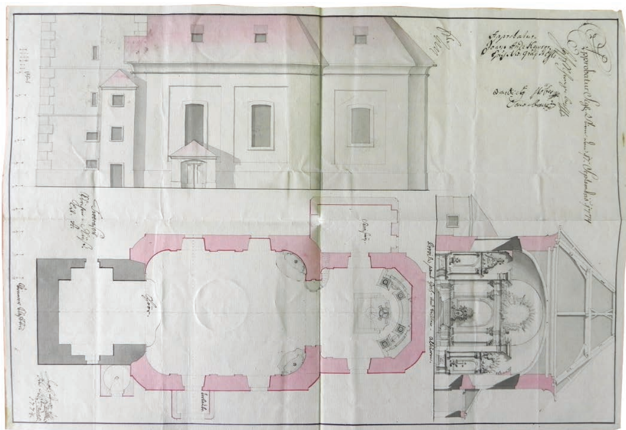
3 – Johann Jobst, návrh přestavby kostela sv. Petra a Pavla ve Svěrázu (panství Český Krumlov), schválený konzistoří a knížetem Josefem I. Adamem ze Schwarzenbergu, 1774. Třeboň, Státní oblastní archiv, pobočka Český Krumlov
