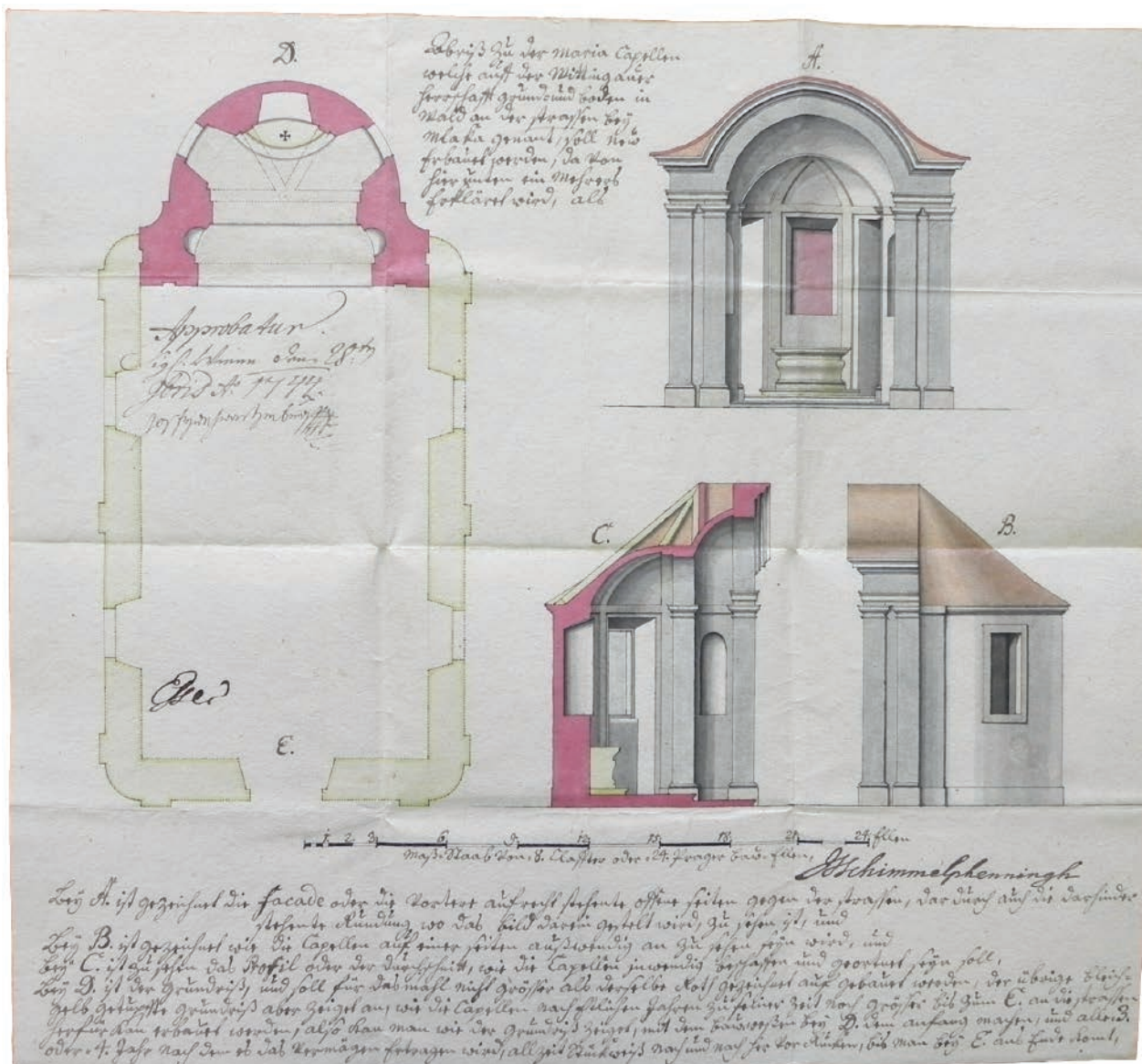
1 – Lorenz Habel, schválený návrh stavby kaple Zasnoubení Panny Marie v Mláče (panství Postoloprty), 1744. Třeboň, Státní oblastní archiv
