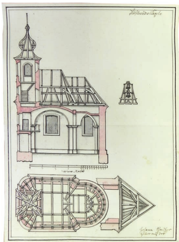
2 – Johann Chadt, návrh krovu nere realizovaného kostela sv. Anny v Počeradech (panství Postoloprty), 1782. Třeboň, Státní oblastní archiv, oddělení Český Krumlov
