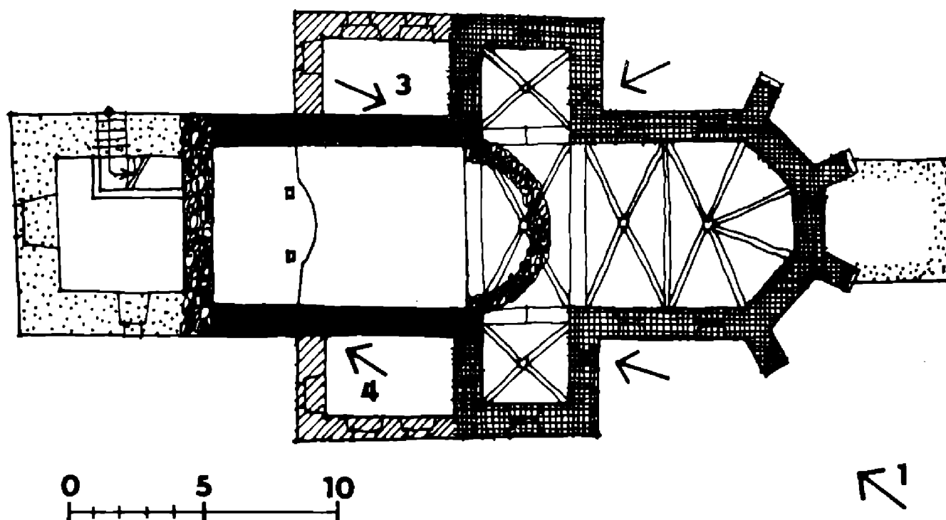
Obr. 2. Kostelec n/Vltavou (okr. Písek), kostel Narození P. Marie, schematický půdorys podle vyobrazení v Soupisu památek... (viz pozn. č. 1, str. 76) s analytickým vyznačením základních stavebních etap. Černě – dochované stěny románského kostela, kroužením doplněn předpokládaný průběh západního a východního ukončení. Křížkovane – raně gotický presbytář a příčná loď, šrafovane – přístavba renesančních empore, tečkovaně – západní věž a východní sakristie. Šipky s čísly označují záběry snímků fotodokumentace, šipky bez čísel umístění druhotně zabudovaných románských oken.
