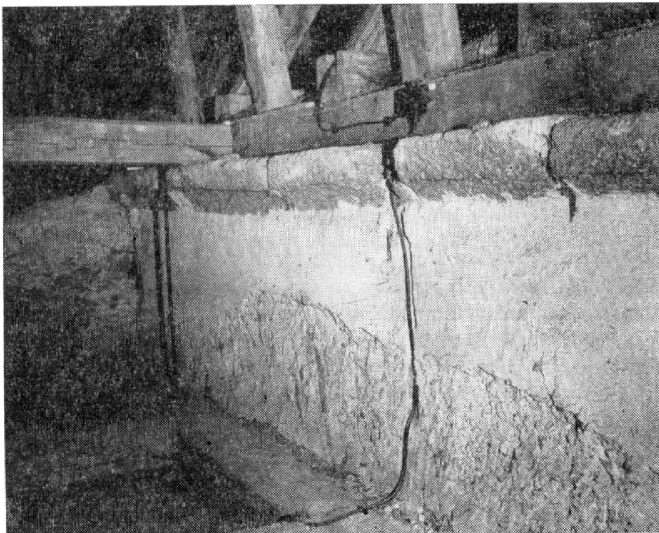
Obr. 3. Kostelec n/Vltavou (okr. Písek), kostel Narození P. Marie, podstřeší nad severní emporou. Pohled k východu podél horní části románské severní stěny lodi. Na koruně zdiva jsou díly tesané řimsy, jejíž fabionový profil končil v místě, kde (na vzdálenějším konci stěny) přiléhá neomítané zdivo nad raně gotickým transeptem. Spodní část viditelného úseku románské stěny je rozrušena vybouráním arkády renesanční empory.
