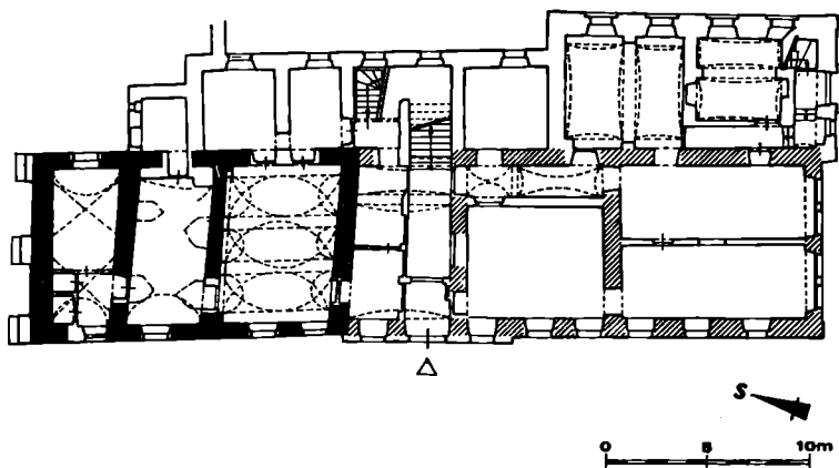
Obr. 19. Čkyň — půdorys přízemí dnešního zámku s dochovanými substrukcemi starší renesanční a barokní stavby.
