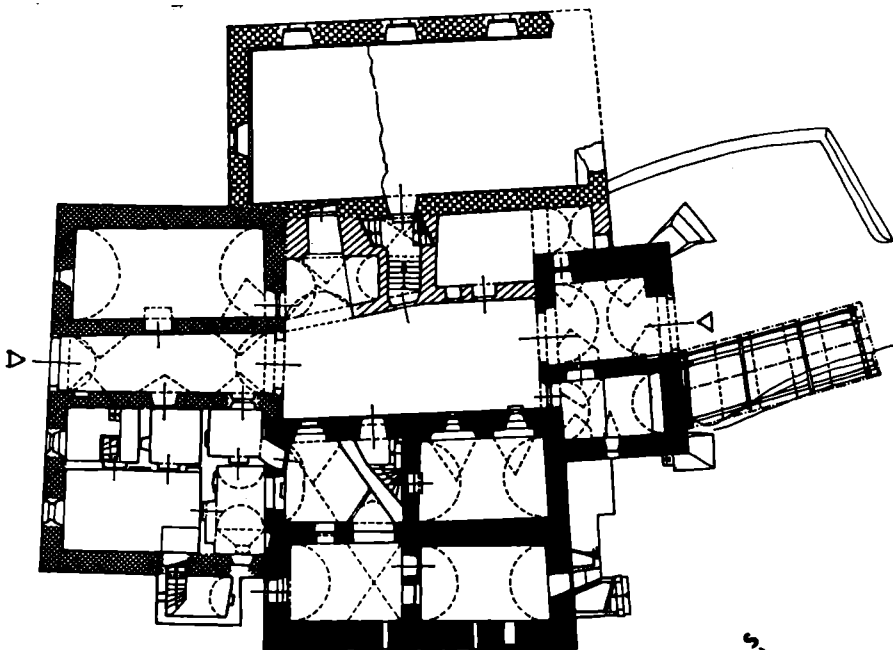
Obr. 13. Dralovice — půdorys přízemí bývalé tvrže.
