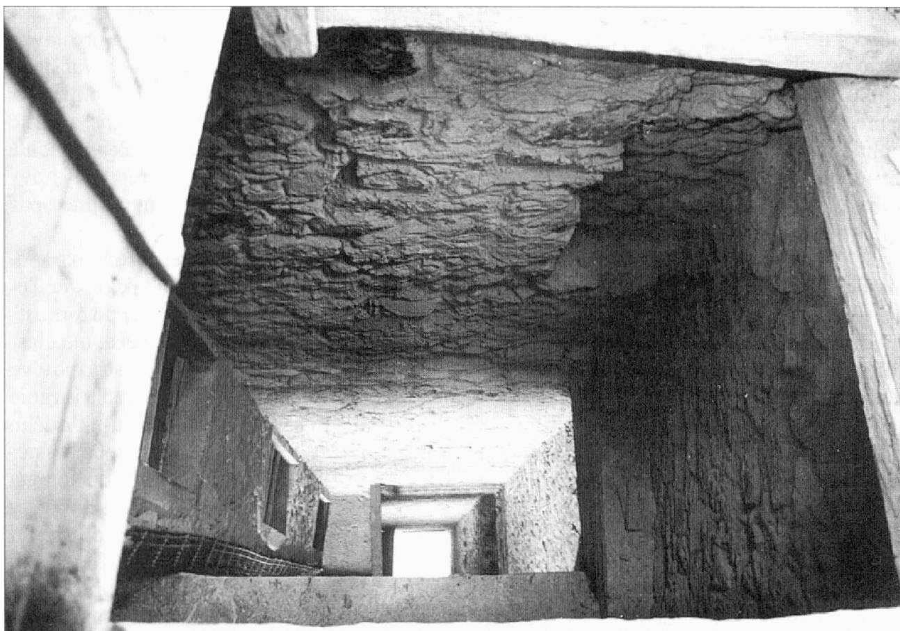
Obr. 5. Šachta rumpálu.
