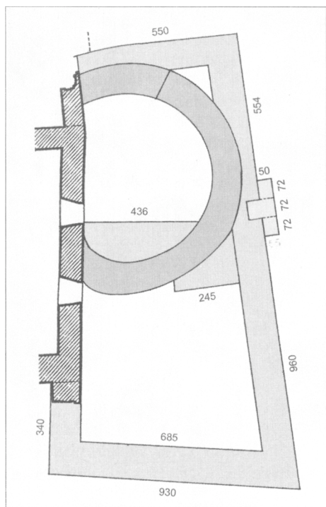
Obr. 4. Borša. Pôdorys okrúhlej stavby a JZ nárožnej veže. Kresba J. Chovanec.
