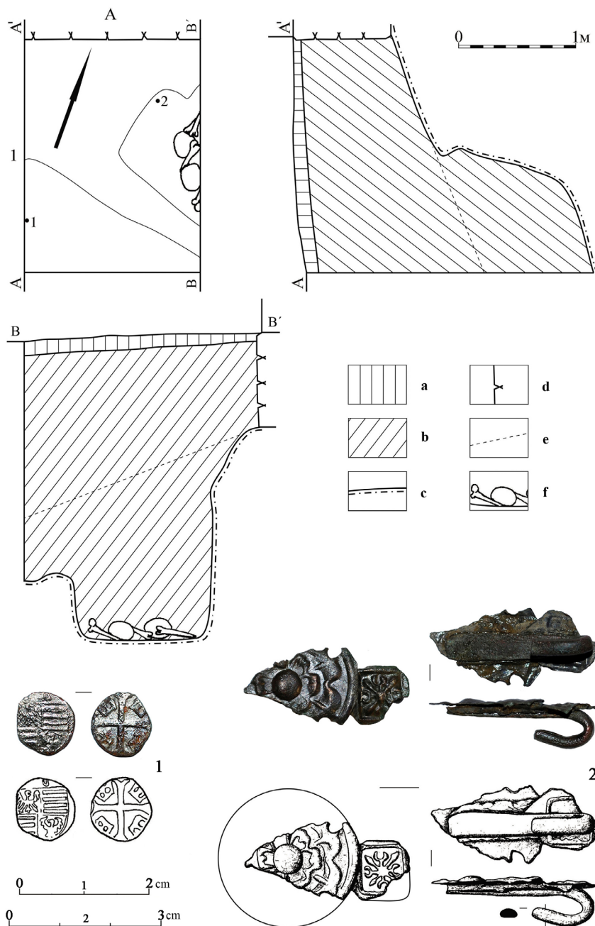
Obr. 25. Stredoveký kostol v Palad' Komariwci. Pôdorys a profil rezu 2 a nálezy z neho. a – povrchová vrstva šedej farby, b – piesok svetlohnedej farby zmiešaný so stavebnou sut'ou a kosťami, c – podložie, d – základ kostola, e – pravdepodobný horizont podložia do doby výkopov v stredoveku, f – ľudské kosti.
