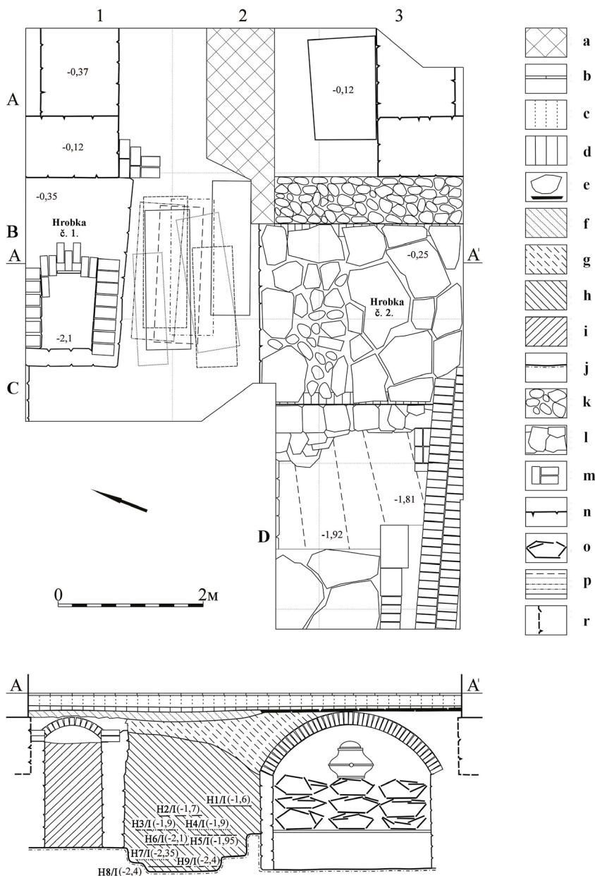
Obr. 6. Stredoveký kostol v Palad Komariwzi. Plán sondy I, pôdorys a profil. a – neskúmaná plocha, b – podlaha, dlažba, c – cementový poter, d – rovnomerná svetlohnedá hlina, e – kamenné dosky, f – stavebná suť, g – piesok so stavebnou suťou, h – svetlohnedý piesok, i – tmavohnedá vrstva s rozptýlenou stavebnou suťou, j – podložie, k – kamenná dlažba, l – murivo z lomového kameňa, m – tehla, n – obrysy kamenného muriva, o – drevené rakvy, p – obrysy hrobových jám, r – pravdepodobné obrysy základov kostola.
