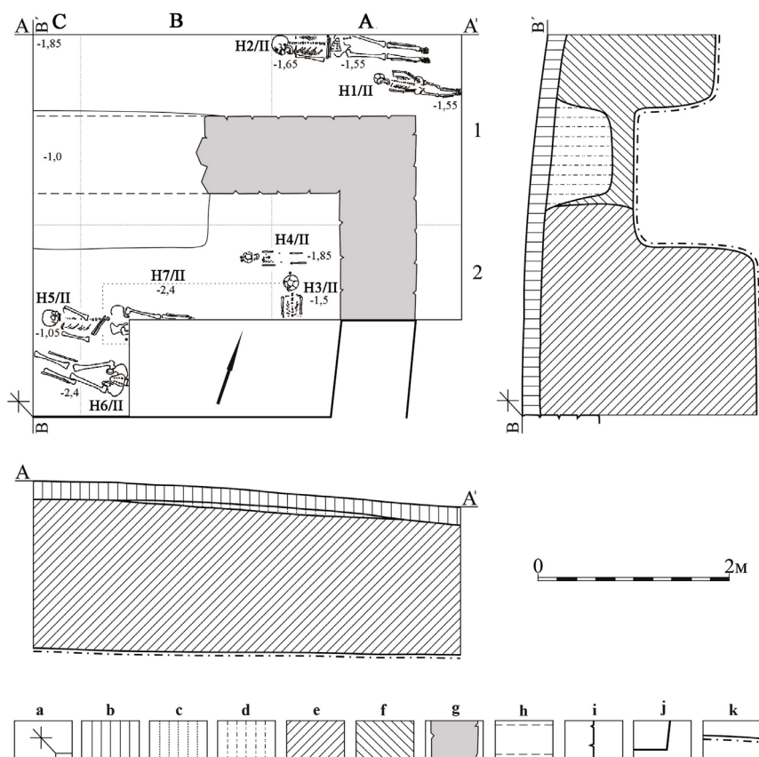
Obr. 16. Stredoveký kostol v Palad' Komarivci. Pôdorys a profily sondy II. a – nivelácia, b – povrchová vrstva šedej farby, c – vrstva stavebnej suty, d – tmavá pôda so stavebnou suťou, e – piesok svetlohnedej farby zmiešaný so stavebnou suťou a kosťami, f – tmavohnedý piesok, g – základ sakristie, h – pravdepodobné obrysy základu sakristie, i – základ presbytéria, j – obrysy súčasných múrov kostola, k – podlažie.
