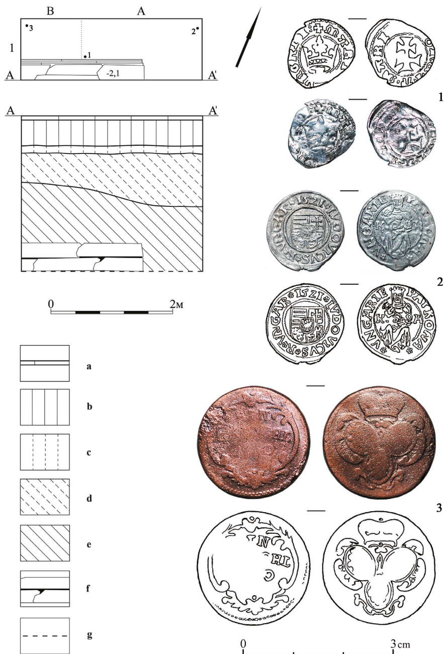
Obr. 14. Stredoveký kostol v Palad' Komarivci. Pôdorys a profil rezu 1 a nálezy z neho. a – podlaha kostola, b – cementový poter, c – rovnomerná svetlohnedá hlina, d – stavebná suť, e – piesok so stavebnou suťou, f – dosky, g – skúmaná úroveň.
