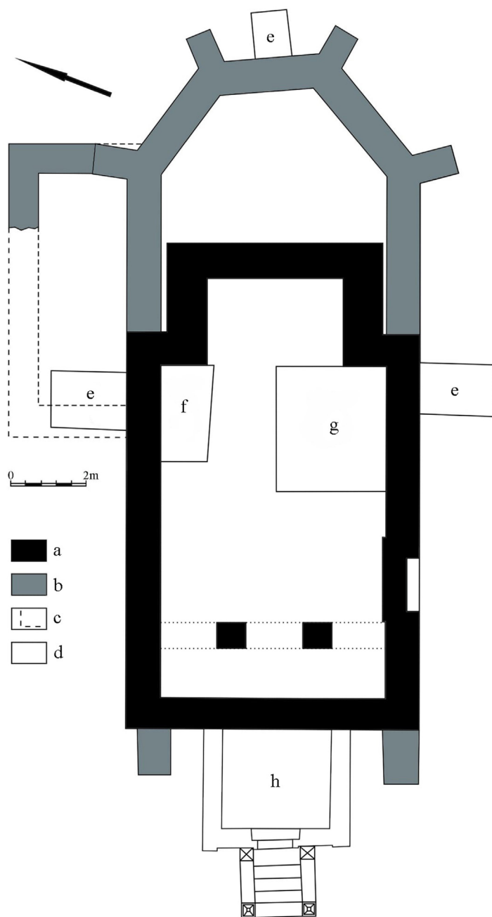
Obr. 28. Stredoveký kostol v Palad' Komarivci. Pôdorys kostola s vyznačením základných stavebných etáp. a – románske obdobie (prelom 13. a 14. storočia), b – neskorostredoveké obdobie (15. storočie), c – predpokladaný priebeh muriva, d – mladšie úpravy, e – po roku 1650 alebo rok 1819, f – rok 1575, g – rok 1729, h – po roku 1791.
