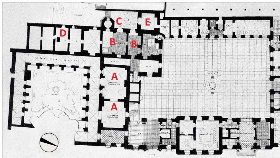
Obr. 1. Nová radnice v Brně – výřez půdorysu přízemí bývalého dominikánského kláštera a zemské soudnice. A – kapitulní síň, B – místnosti pro ukládání stavovských písemností, C – polygonální schodišťový přístavek, D – prostory technického mezipatra nad románským refektářem, E – přístavba pro záchody z doby po roce 1629. Podle Dřímál 1947, upravila J. Janišová, 2025.
