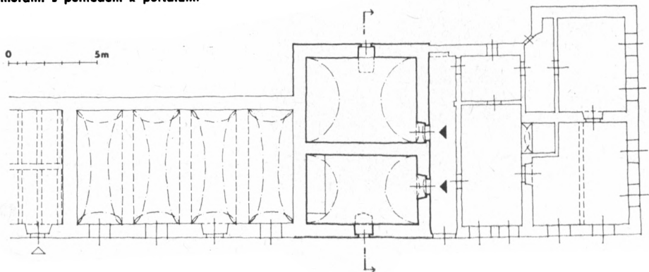
Obr. 22. Solopysky (PB) čp. 12. Půdorys obytného stavení. Silněji vytažena pozdně gotická komorová část s původními portály a okny. Nahoře řez komorami s pohledem k portálům.
