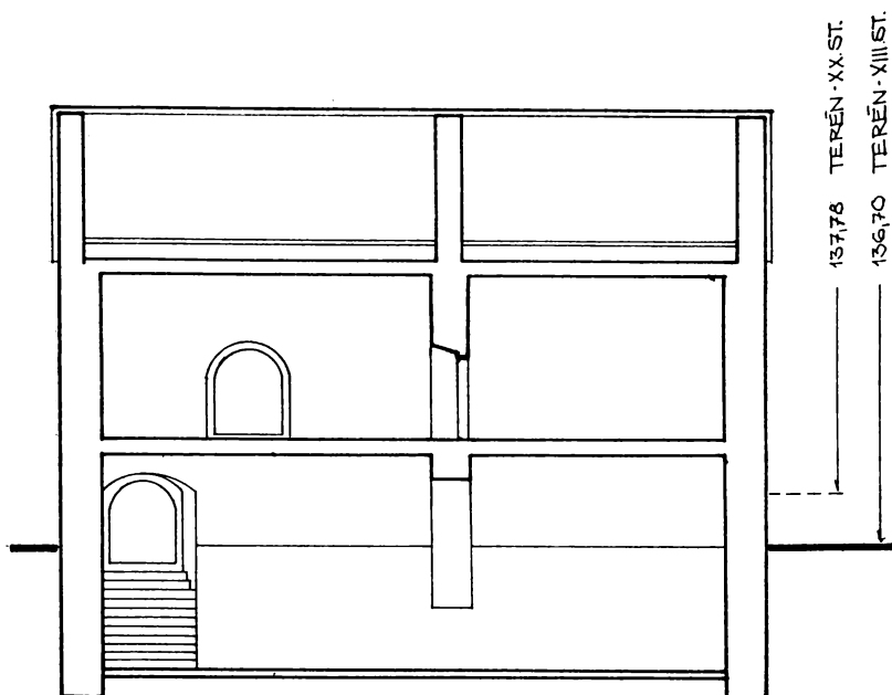
obr. 21. Hypotetická rekonštrukcia domu z 2. pol. 13. st. Pozdĺžny rez západný.
