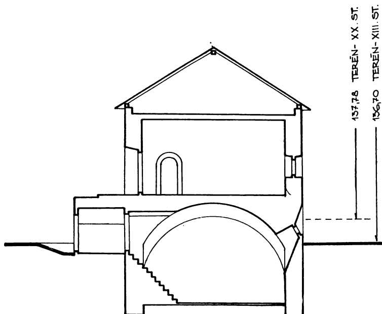
Obr. 20. Hypotetická rekonštrukcia domu z 2. pol. 13. st. Pričný rez severný.
