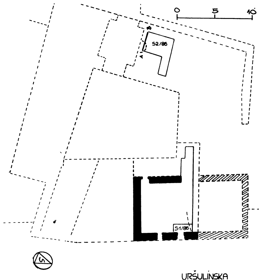
Obr. 1. Uršulínska ul. č. 6 — situácia parcely č. 3, S1/86 a S2/86,
