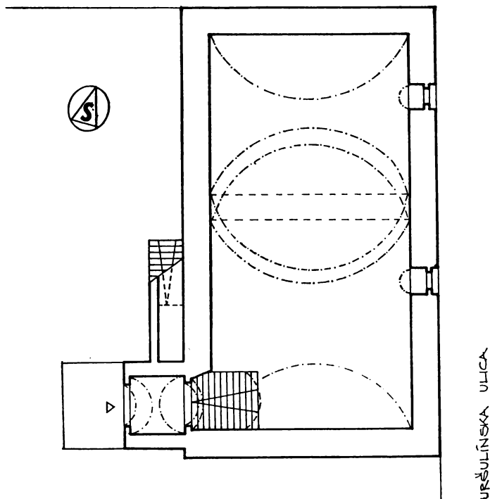
Obr. 18. Hypotetická rekonštrukcia domu z 2. pol. 13. st. Pôdorys dolného podlažia.
