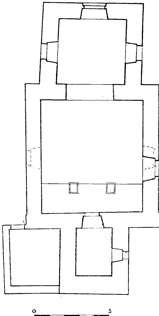
Kostel v Rokytíně. Vyměřil ing. arch. J. Hlyzler.
