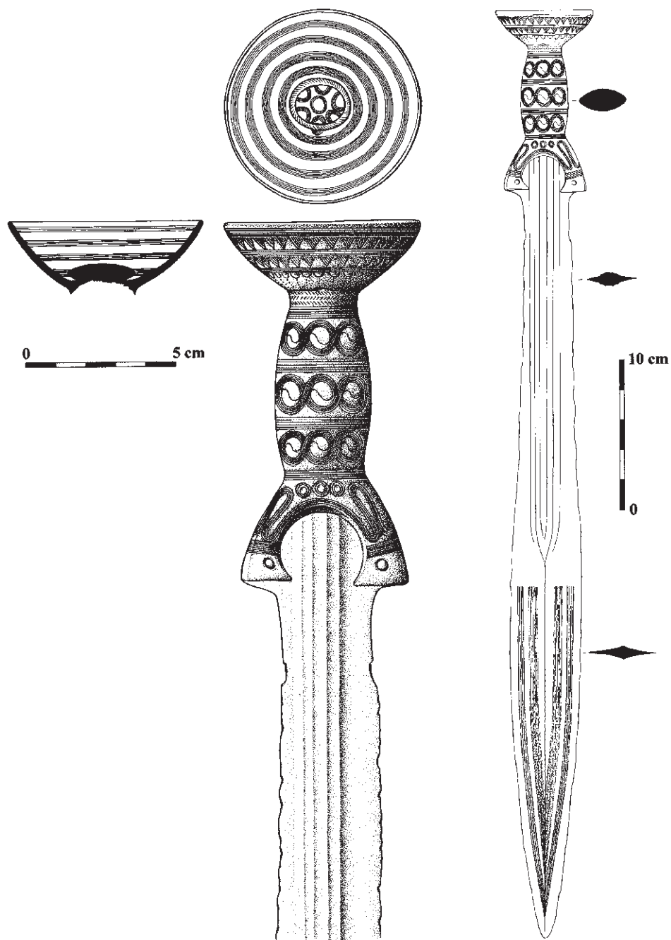
Obr. 2. Brno – Královo Pole, okr. Brno-město. Bronzový meč s číškovitou rukojetí (kresba P. Kos – A. Krechlerová – M. Přichystal).
