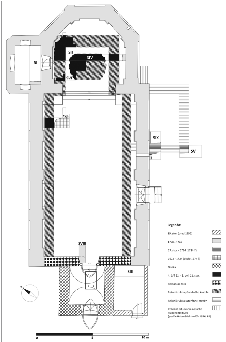
Obr. 9. Hronský Beňadik, Kostol sv. Egidia. Zameranie a slohová analýza. Autori M. Hanuš, M. Haviarová a T. Haviar. Abb. 9. Hronský Beňadik, Kirche St. Ägidius. Vermessung und Stilanalyse. Erstellt von M. Hanuš, M. Haviarová und T. Haviar.
