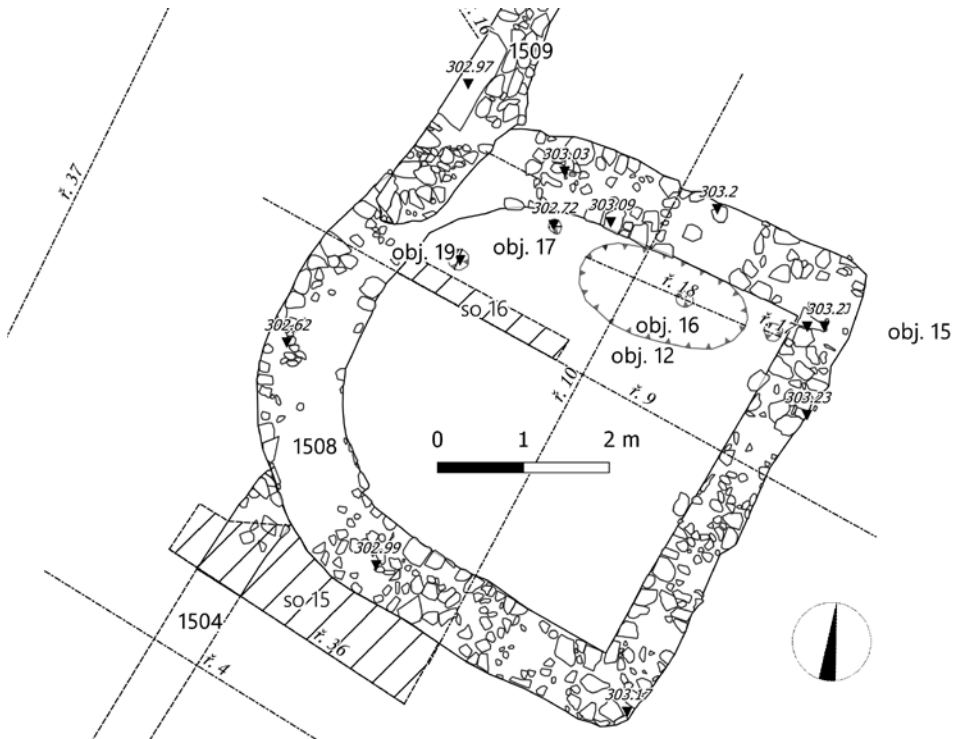
Obr. 5. Púdorys bašty. Vytvořil K. Derner.
