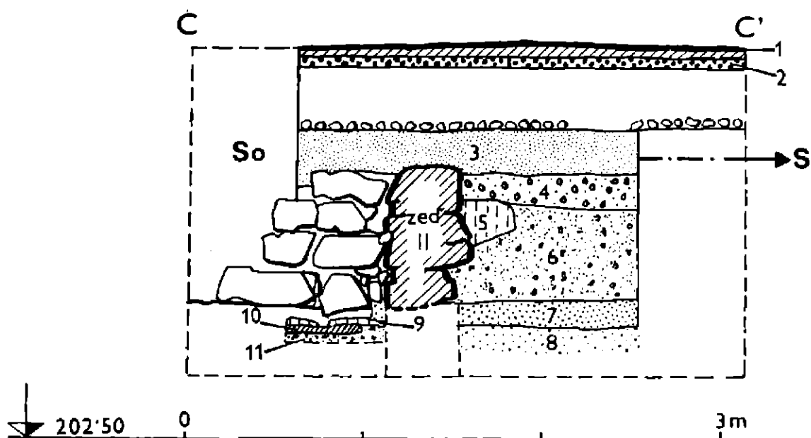
Obr. 3. Praha 9, Vysočany, ul. E. Klímy. a) Podélný řez objektem ve směru SJ; b) V-Z profil: 1, 2 – jílové vrstvy světlé až šedohnědé barvy, 3 – šedohnědá jílová, 4 – šedohnědá písčité vrstva, 5 – spálená hlinitá, 6 – světle hnědý jíl s pískem, 7 – žlutý písek, 8 – tmavohnědý jíl, 9 – jílová pecka, 10, 11 – písek, 12 – žlutý jíl, 13 – kosti, 14 – pískovec. c) S-Z nároží objektu od východu: 1 – asfalt, 2 – dlažba, 3 – písek, 4 – říční valouny, 5 – žlutý jíl, 6 – šterkopísek, 7, 8 – říční písek, 9 – světlý jíl, 10 – pevný šlérk, 11 – rezavý šterkopísek, SO – původní sonda stavbařů. Kresba: V. Huml, J. Steklá.
