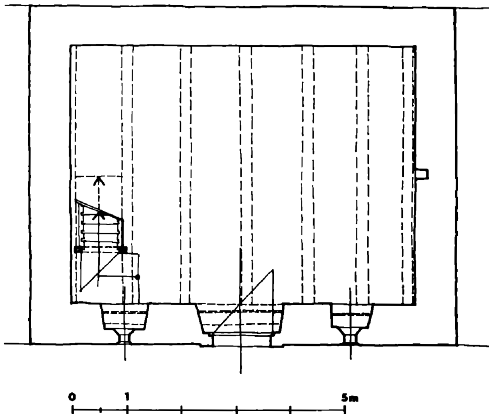
Obr. 3. Koterov žp. 7. Půdorys přízemí sýpky se dvěma křížkovými střílnami ve vstupní stěně.
