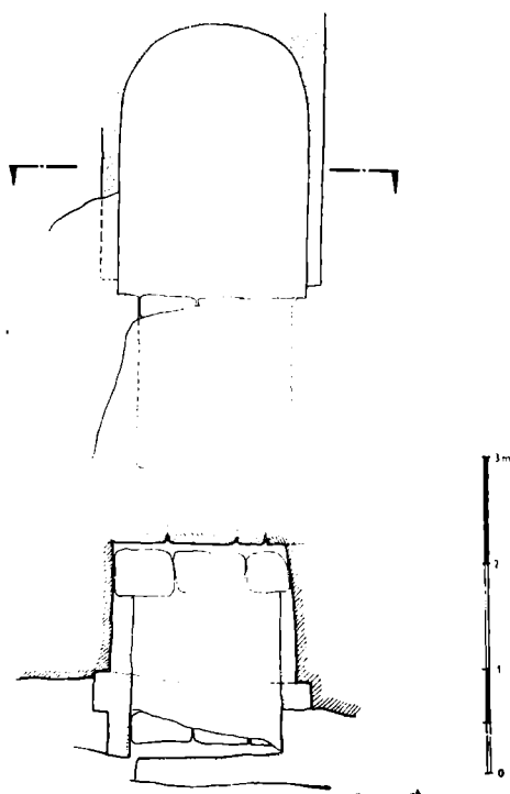
Obr. 2. Hrad Valdštejn, chodba na 2. skalním bloku, pohled a půdorys. Tečkovaním lemovaná linka — sekáním npravená skála. Měřil F. Gabriel, kresba P. Macek.
