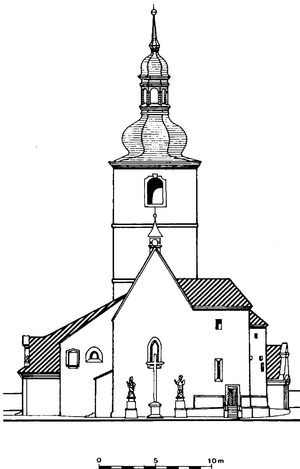
Obr. 10. Východní pohled na kostel sv. Martina v Radomyšli.
