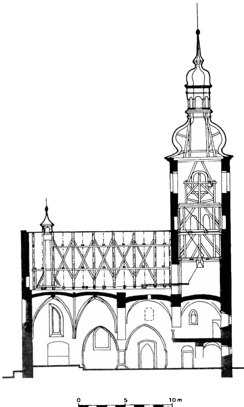
Obr. 13. Podélný řez kostelem sv. Martina v Radomyšli s pohledem k jihu.
