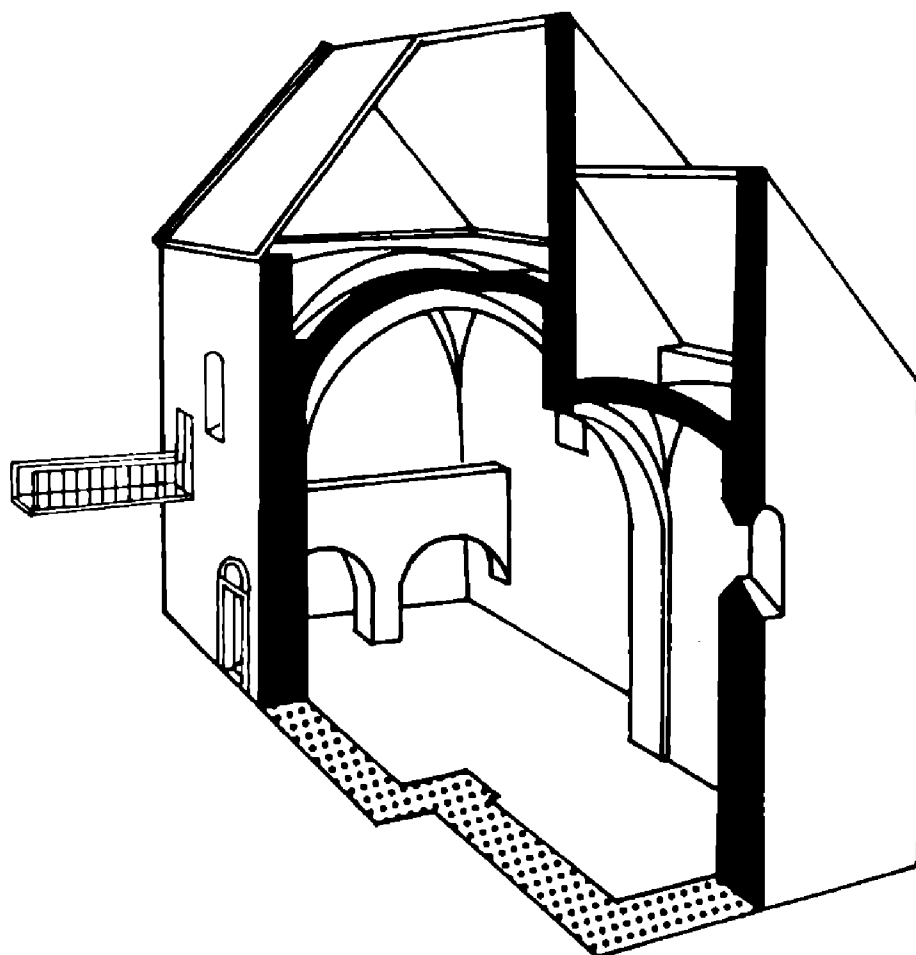
Obr. 14. Rekonstrukce románského kostela – řez s pohledem k panské tribuně – rekonstrukci na základě archeologického a stavebního výzkumu provedl ing. arch. F. Kašíčka ze Státního ústavu pro rekonstrukci památkových měst a objektů.
