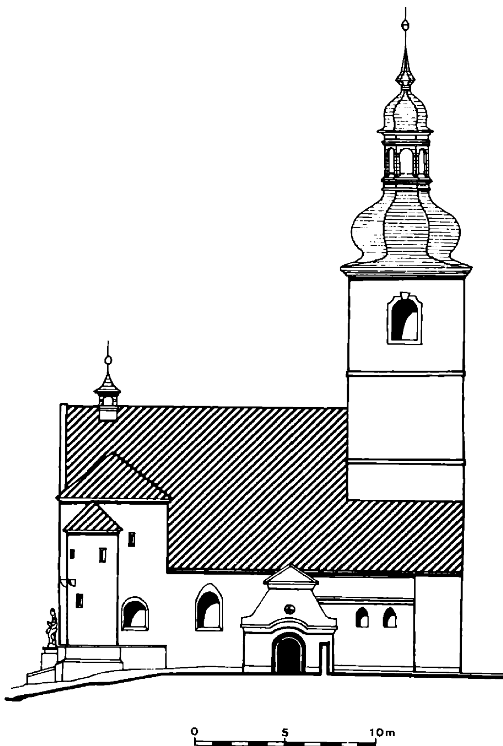
Obr. 11. Severní pohled na kostel sv. Martina v Radomyšli.
