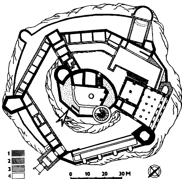
Obr. 2. Bojnice – hrad, situácia hradu so stavebnou etapizáciou podľa D. Menclovej a s označením Archívneho krídla (1 – koniec 13. stor.–zač. 16. stor.; 2 – 2. pol. 16. stor.; 3 – pol. 17. stor.; 4 – 19. stor.). Kresba M. Bóna.
