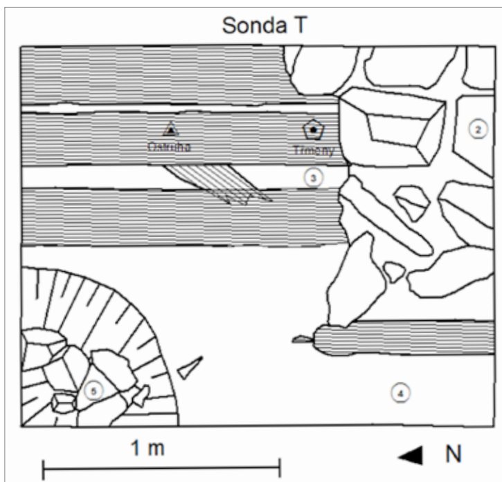
Obr. 21. Zámeček, k. ú. Stráž. Sonda T, úroveň spálené dřevěné konstrukce. Vyznačena místa nálezů třímení a ostruhy. Kresba F. Kasl, 2019.
