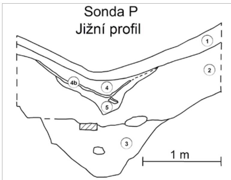
Obr. 24. Zámeček, k. ú. Stráž. Sonda P, jižní profil. 1 – svrchní půda; 2 – písčitá vrstva s kameny (zloмок keramiky doby bronzové); 3 – jílový sediment, ve spodní části s hlinitou příměsí, s kameny a kusy ohořelých jedlových dřev (na rozhraní vrstev 2 a 3 trámeček, z něhož byl odebrán vzorek č. 3 na C14, vzorek č. 4 odebrán z jedlového dřeva u dna příkopu); 4, 4b, 5 – kompaktní souvrství s kameny; 4b – uhlíky s popelem. Kresba F. Kasl, 2019.
