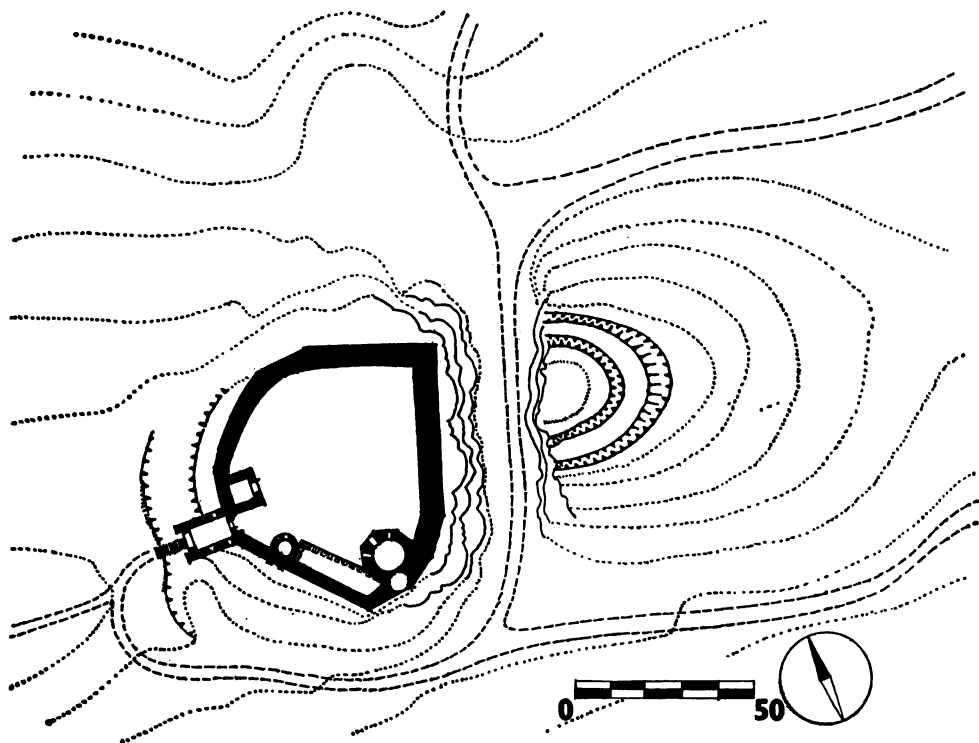
Obr. 2. Schéma staršího předsunutého valového opevnění před Novým hradem.
