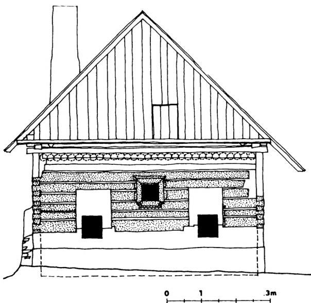
Obr. 3. Lučice čp. 2 (okres Klatovy), štítové průčelí domu. Tečkované jsou značeny dochované části původní roubené konstrukce domu ze 16. století, černě původní okenní otvory (u spodních oken doložené stopami zárubní), čárkovaně průřez povalového stropu (zachovaného v zadní polovině místnosti) a předpokládaná úroveň původní podlahy.
