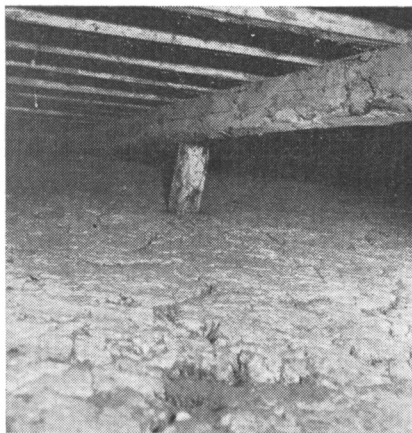
Obr. 4.–5. Krnín čp. 3 (okr. Český Krumlov). Izolační dřevohlíněná konstrukce (lepenec) v podstřeší zadní patrové komorové části pozdně gotického domu – usazení krokvi, nesoucích bednění a mazaninu, na roubeném věnci, a pohled vzhůru ke hřebeni střechy mezerou mezi vnějším lícem hlíněné izolace a vrchním krokem s krytinou.
