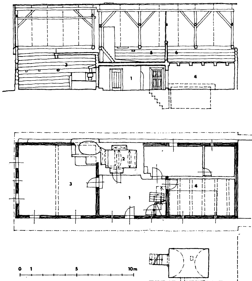
Obr. 1. Lučice čp. 2 (okres Klatovy), půdorys přízemí se sklepem (dole) a podélný řez (nahoře). V půdorysu jsou šrafovány roubené stěny původní výstavby domu ze 16.–17. století. 1 – vstupní síň v přízemí, 2 – mladší zděná černá kuchyně, 3 – obytná místnost s dochovanou polovinou původního pavalového stropu, 4 – spodní komora, 5 – dnešní horní síň s původním portálem do horní komory, 6 – zbytek horní komory.
