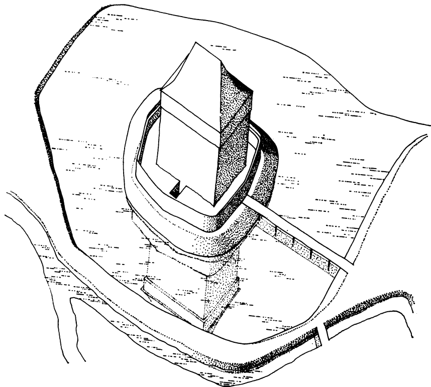
Obr. 5. Hlubany. Rekonstrukce tvrze v nadhledové axonometrii, provedená lineární kresbou se stínováním.
