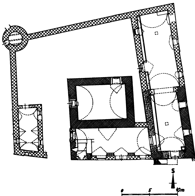
Obr. 4. Kestřany — půdorys přízemí Dolní tvrze ve stavebně historické analýze, stav 1986. Husté a řídké mřížky značí 2 gotické stavební fáze, ostatní zdivo je renesanční a mladší. (F. Kašíčka)
