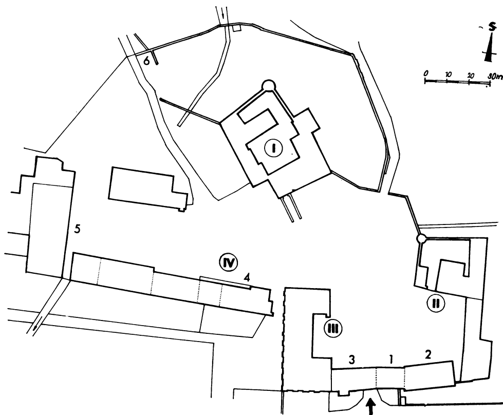
Obr. 1. Kestřany — celková orientační situace souboru: I. Horní tvrz, II. Dolní tvrz, III. zámek, IV. hospodářský dvůr. 1 — středověká hospodářská budova, 2 — bývalá renesanční sladovna, 3 — renesanční budova dnešních stájí, 4 — bývalá ratejna a vepřín, 5 — barokní stodola, 6 — horní brána. (F. Kašička)
