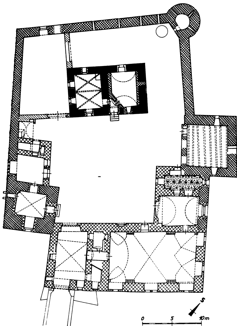
Obr. 2. Kestřany — půdorys přízemí Horní tvrze ve stavebně historické analýze, stav r. 1986 — vybouření dodatečných příček a mezistropů. Černé značeno raně gotické zdivo „purkrabství“ husté a řídké mřížky značí 2 pozdější gotické fáze, ostatní zdivo je renesanční a mladší. (F. Kašíčka)
