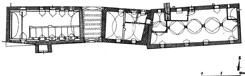
Obr. 6. Kestřany – přední hospodářské budovy, půdorys přízemí ve stavebně historické analýze. Šikmé mřížky značí zdívo gotické, mřížky kolmé ke konstrukci – renesanční, ostatní mladší. Přerušovaná šrafura označuje zařazení hypotetické. (F. Kašíčka)
