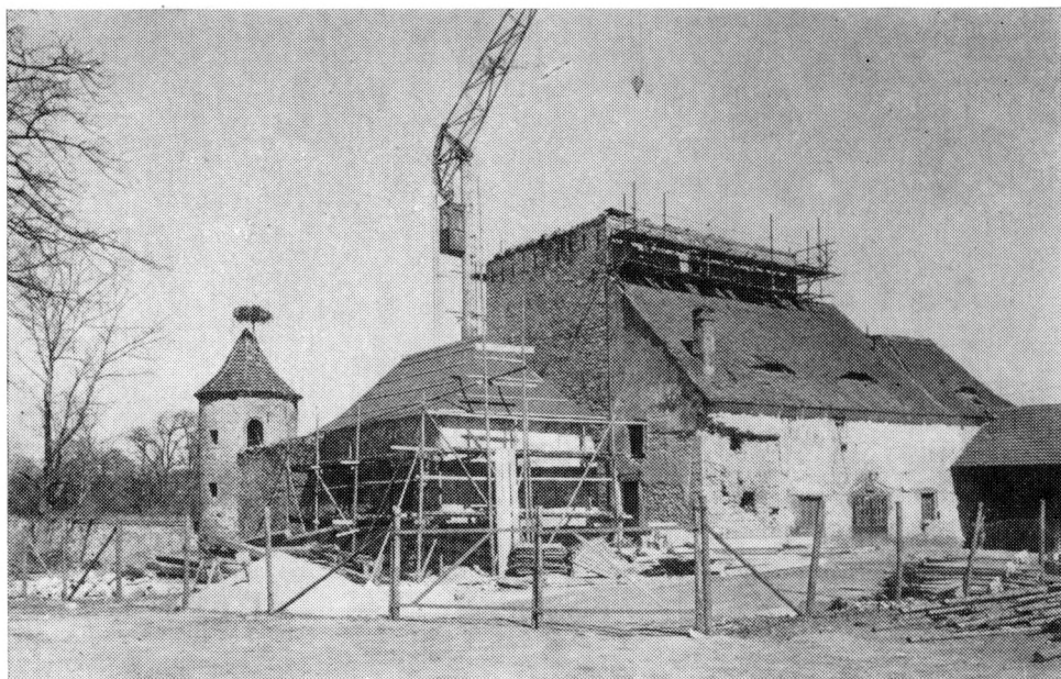
Obr. 10. Kestřany — Dolní tvrz v průběhu zabezpečovacích prací. (Foto V. Uher)
