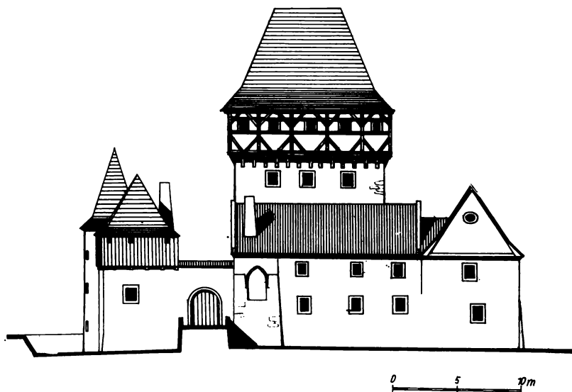
Obr. 5. Kestřany – čelní průčelí Dolní tvrze před započatím zabezpečovacích prací a rekonstrukce po-doby v 16. stol. (F. Kašíčka)
