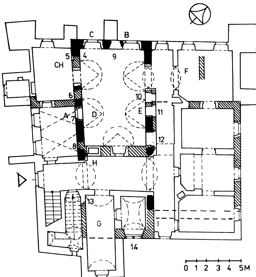
obr. 3. Bratislava — Devín, kaštieľ na Hutníckej ul. č. 25. Pôdorys prízemľa, stavebno-historická analýza. Čierne murivo I. etapy, šrafované murivo II. a III. etapy, 4. ostenie okna z I. etapy, 5. okno z III. etapy, 6. otvor z II. etapy, 7. portál z III. etapy, 8. vetrací otvor z I. etapy, 9 až 12, otvory z III. etapy, 13. portál z III. etapy, 14. okno s paspartou z III. etapy. Písmenami A—I sú označené archeologické sondy.
