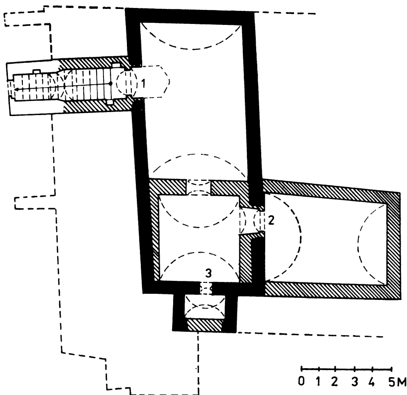
obr. 2. Bratislava — Devín, kaštieľ na Hutníckej ul. č. 25. Pódorys suterénu, stavebno-historická analýza. Čierne murivo I. etapy, šrafované murivo II. a III. etapy. 1. vstupný portál z III. etapy. 2. vstupný portál z II. etapy. 3. vstupný otvor z I. etapy.
