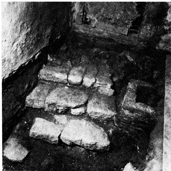
Obr. 5. Bratislava — Devín, kaštieľ na Hutníckej ul. č. 25. Portál (7) z III. etapy so schodiskom odkrytým v AS A.
