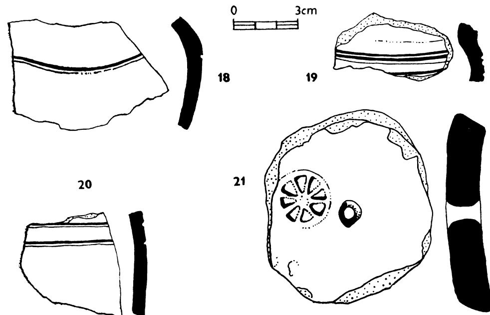
Obr. 10. Výběr keramiky ze s. IV, V a IX z 1. pol. 13. stol. (obj. 1 – 3, 4, 6, 14 a 16; obj. 3 – 1, 15; obi. 7 – 2, 5, 7, 8, 10, 11 a 12, hl. 160–170 cm). Kreslíla: K. Scheuflerová.
