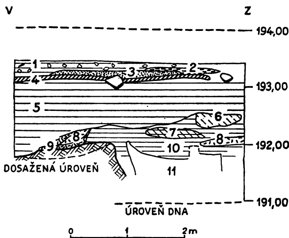
Obr. 4a. Sonda IX (1985), řez V-Z. 1 – hnědá hlína s opukovými zlomky a částmi cihel, 2 – okrová malta, 3 – zlomky cihel, 4 – černá hlinitá vrstva se zuhelnatělým dřevem, 5 – hnědý jíl se zl. opuky, mazanici zl. uhlíků, 6 – šedohnědá břidlice, 7 – hnědý jíl, 8 – šedohnědý jíl s uhlíky, 9 – červeno-hnědá mazanice, 10 – černá hlína s uhlíky, 11 – tmavě šedá hlína s jílem, zl. dřevěných částí – pec, 12 – výplň objektu č. 7: tmavě šedá hlína s jílem a uhlíky.
