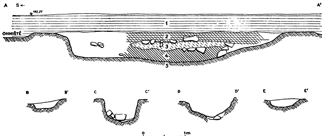
Obr. 8b. Obj. 9 (frez S-J): 1 – hnědá hlína s uhlíky, štěrků opuky, 2 – šedohnědá hlína, 3 – červeno-žlutý jíl s mazanicí a kameny, 4 – tmavě šedá hlína s keramikou 13. stol. Kreslil: V. Huml.
