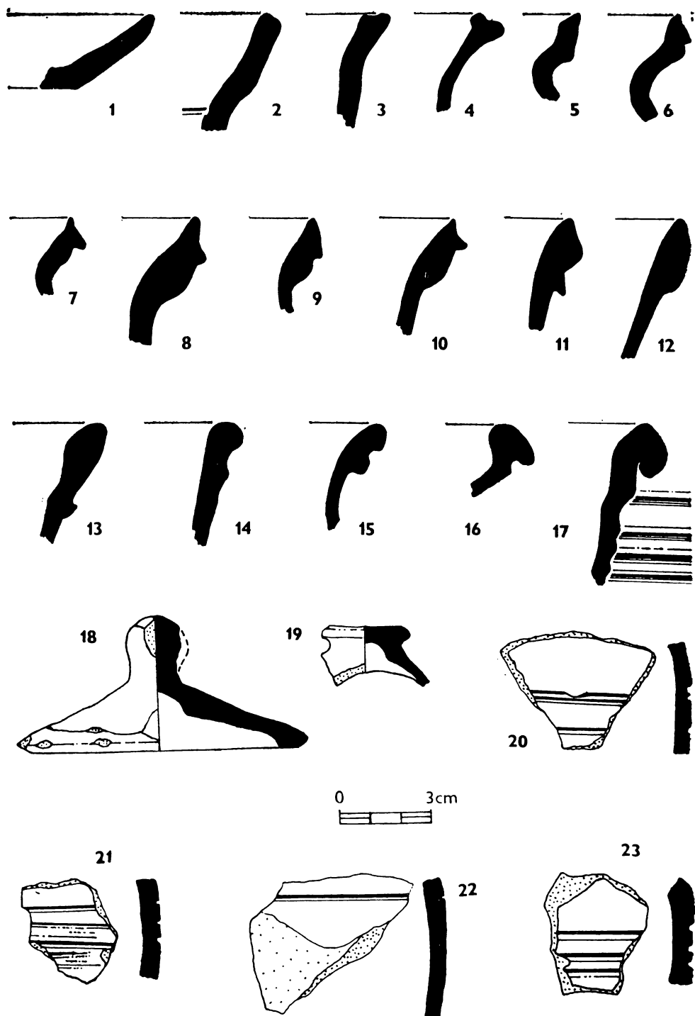
Obr. 9. Výběr keramiky ze sondy IV, V a IX z 1. pol. 13.–16. stol. (obj. č. 1 – 17; obj. 3 – 15, 19, hl. 130 až 150 cm; obj. 7 – 1, 2, 9, 13, 14, 16, 18, 20, 21 až 23). Kreslíla: K. Scheutlerová.
