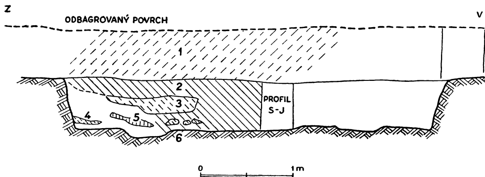
Obr. 8a. Obj. 9 (frez V-Z): 1 – hnědý jíl s opukovými zlomky, uhlíky, 2 – šedá hlína s uhlíky, 3 – žlutý jíl s mazanicí, 4 – žlutý jíl, 5 – popel světle růžové barvy, 6 – světle šedá ssuť.
