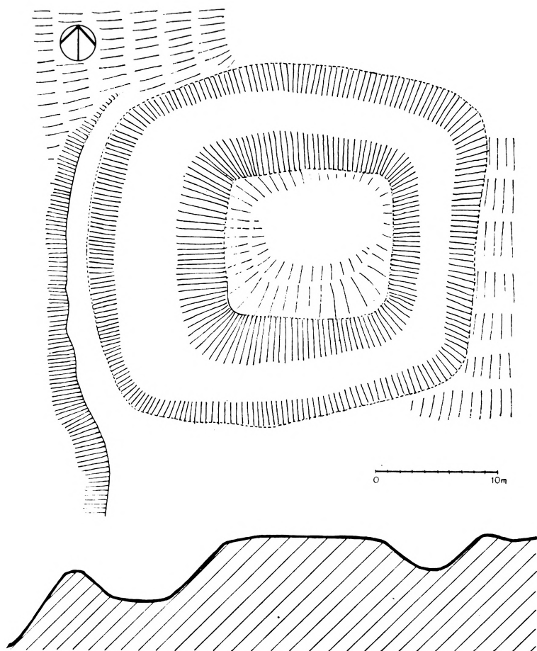
Obr. 2. Solec. Púdorys tvrziště a řez. Zaměření autor.
