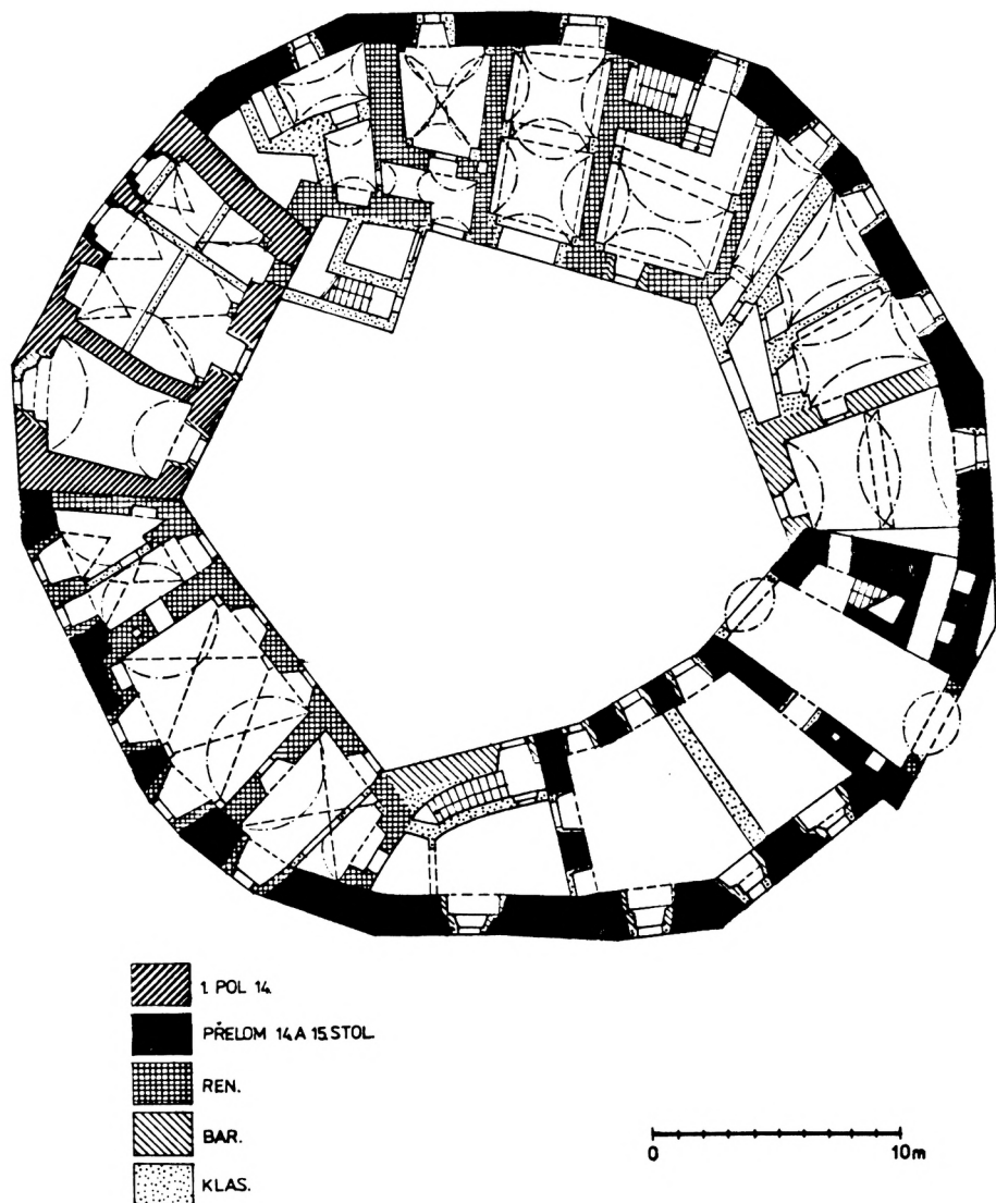
Obr. 6. Nepomyšl. Půdorys přízemí s vyznačením stavebního vývoje podle H. Soukupové.
