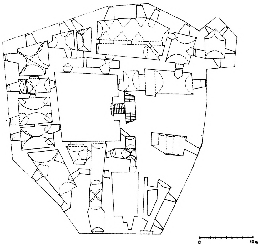
Obr. 11. Chanovice. Půdorys přízemí zámku podle zaměření stavební fakulty ČVUT Praha.
