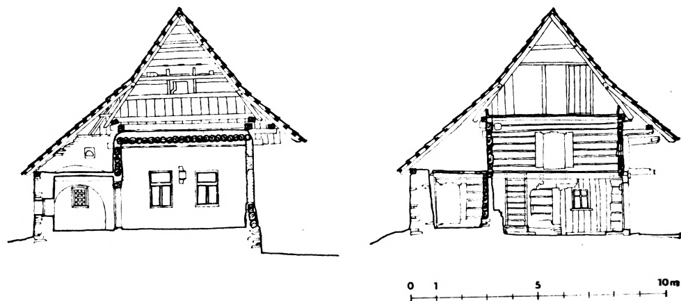
Obr. 5. Čistá čp. 171, příčné řezu jizbou (vlevo) a třetím dílem půdorysu. Zaměření a kresby J. Svrový a autoři, 1988.
