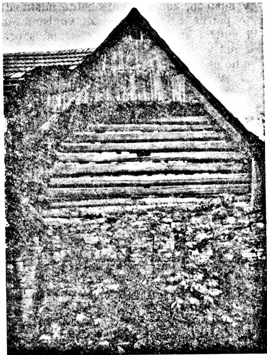
Obr. 7. Čistá čp. 109(†), zadní štít domu v patře s roubenou komorou, jejíž část vsunutá do krovu byla uzavřena roubenou poloklenbou. Foto J. Škabrada, 1988.
