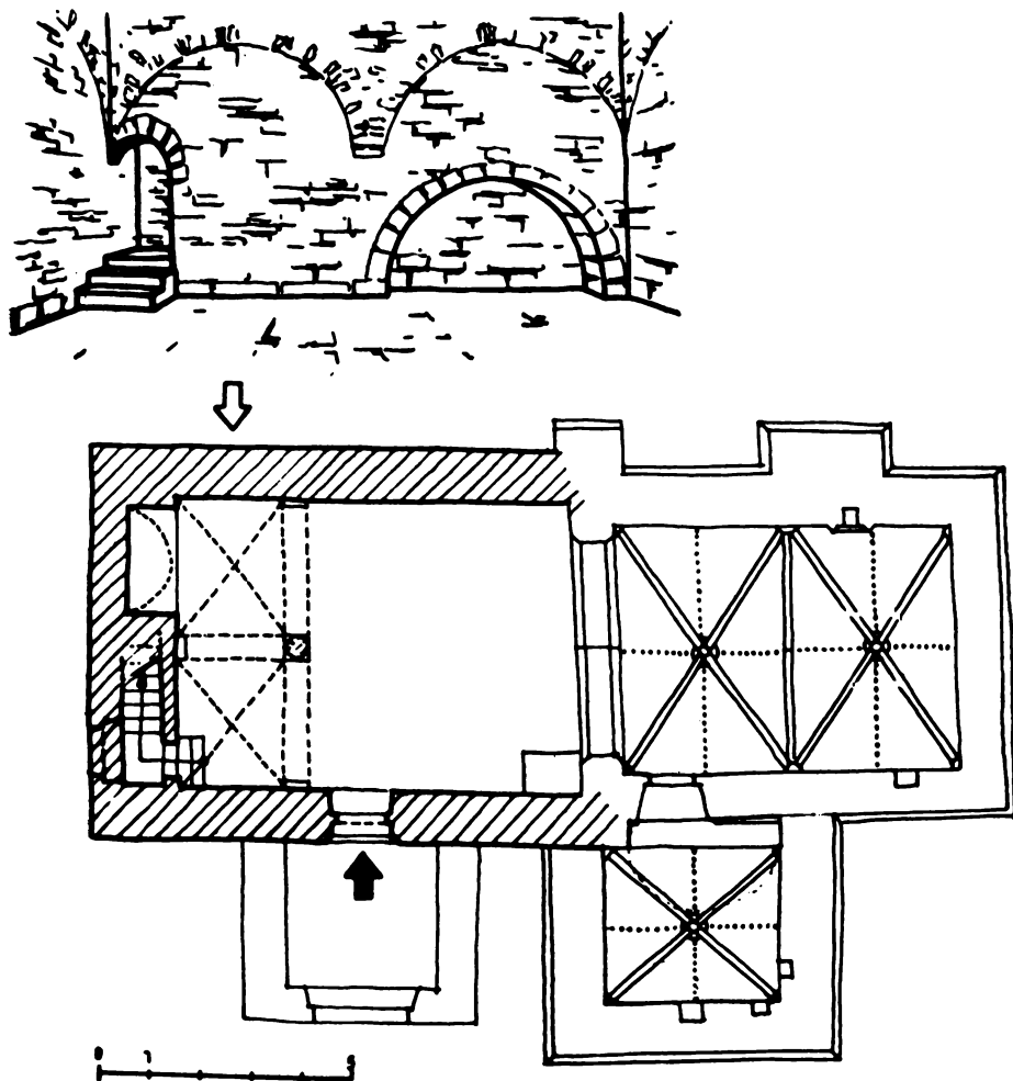
Obr. 2. Půdorys kostela sv. Jakuba v Bedřichově Světcí ze zač. 13. stol. a perspektivní pohled na stěnu pod tribunu (M. Radová).
