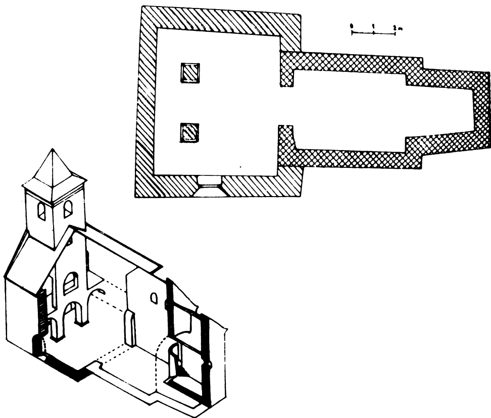
Obr. 4. Kostofany p. Tr., půdorys zděného kostela z 1. pol. 11. stol. s přístavbou západní tribuny ze 13. stol. (podle V. Mencla).
