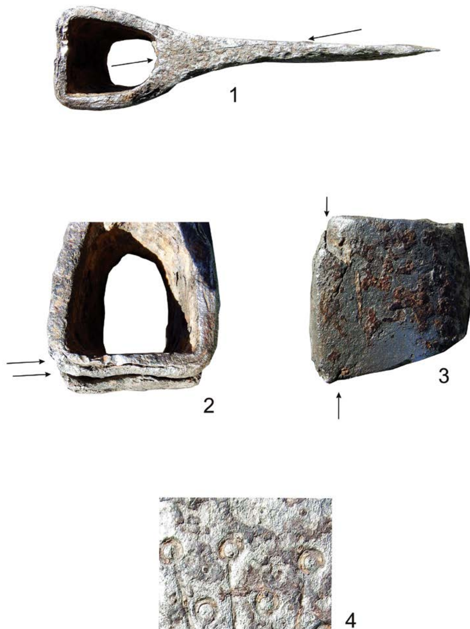
Obr. 4. Staré Jesenčany (okr. Pardubice). Technologické stopy. 1) šipky zvýrazňují průběh sváru mezi listem a ohybem oka; 2-3) šipkami je zvýrazněn průběh svárů opravy prasklého oka (?) a přivařené zesílené plošky týla. 4) detail výzdoby. Foto J. Musil
