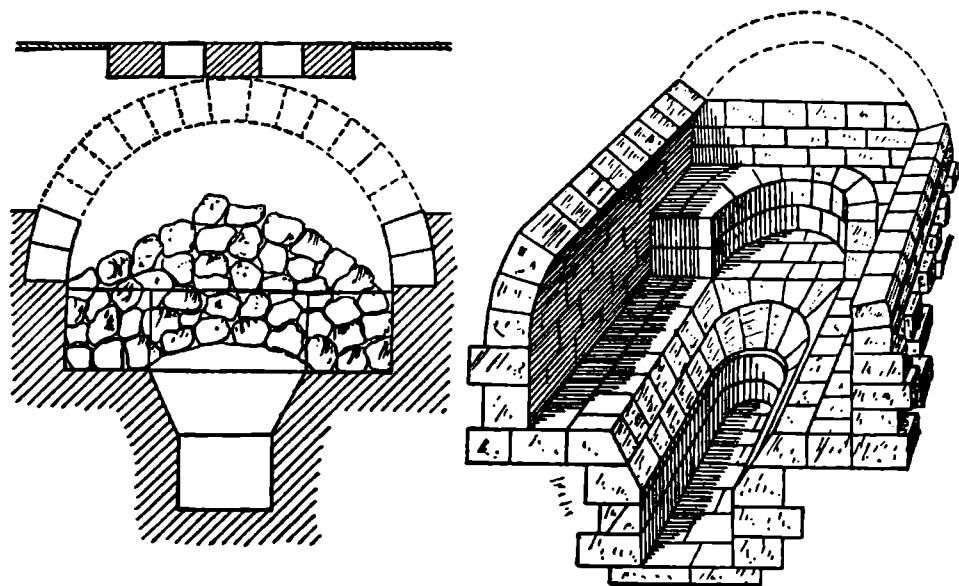
Abb. 4. Marburg, BRD. Warmlufttheizanlage im Schloss
