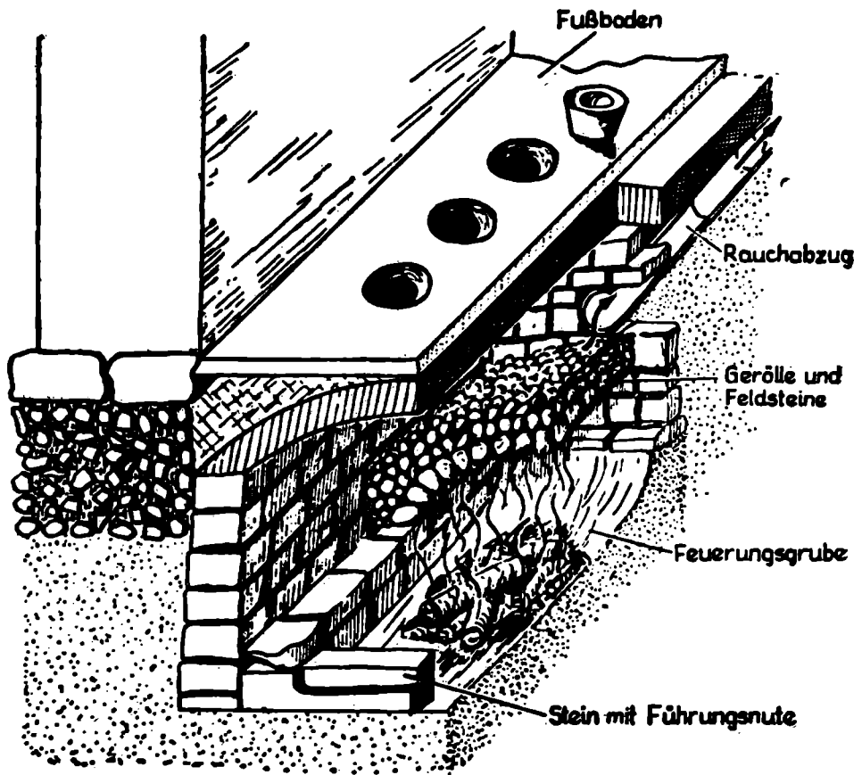
Abb. 2. Altmühlhausen, DDR. Rekonstruktion der Steinofen-Luftheizung in dem Komturensitz. (Nach H. J. Barthel)
