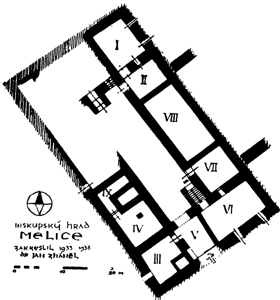
Abb. 1. Melice bei Vyškov. Grundriss der Burg. I — Schlafzimmer des Burgkaplans, II — Kammer?, III — Wachstube, IV — Küche?, V — Burgeinfahrt, VI — Keller, VII — Vorratskammer, VIII — Kammer?, IX — Stiegenhaus. SW von I liegt die Burgkapelle. (Nach J. Zháněl)
