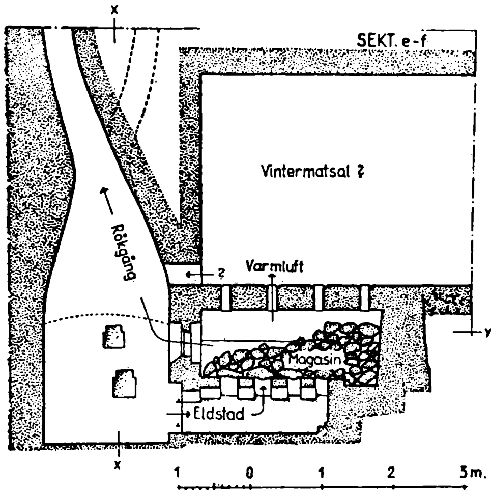
Abb. 3. Vadstena, Schweden. Rekonstruktion einer Heizanlage
