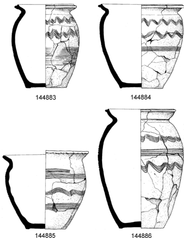
Obr. 201 – Výzkum R15. Keramické nádoby náležící k nadzemnímu objektu O28/R15. Kresba A. Šik.
