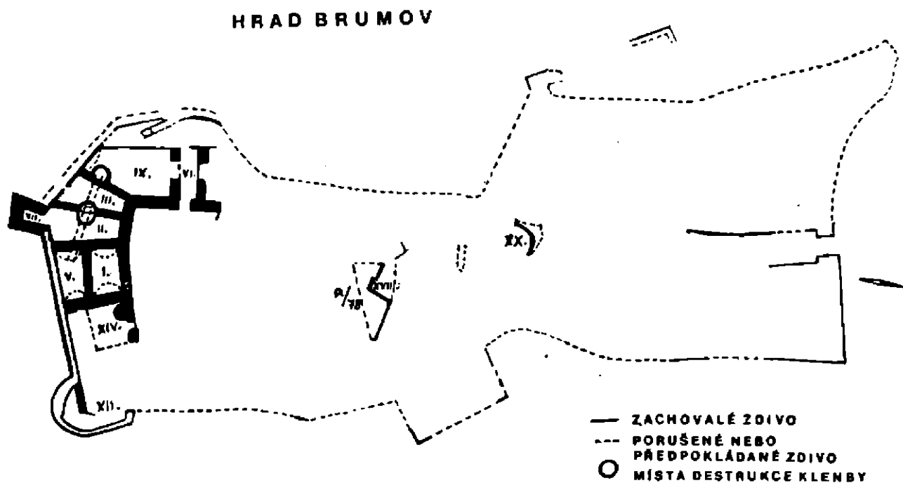
Obr. 1. Schématický náčrt půdorysu hradu Brumova podle předběžného zaměření Ing. Z. Ptáčka (stav po výzkumu v r. 1978). Přibližné měřítko 1:100.
