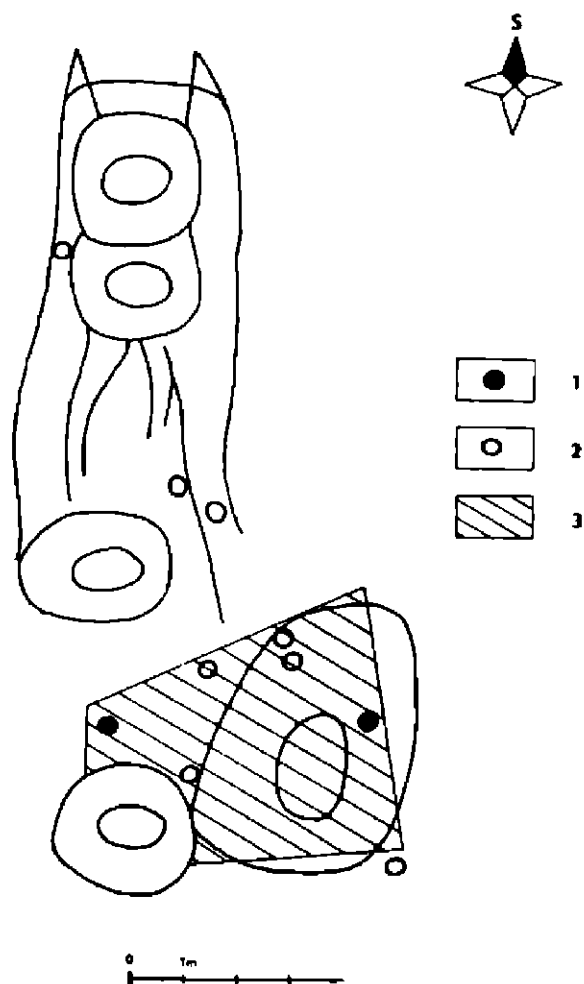
Obr. 3. ZSO Potálev, okres Tábor. Průzkum minohledačkou Mi W 3 P. 1 - Předpokládaná místa nálezů kovů, 2 - anomálie, projevující se hlubším tónem, 3 - anomálie v ploše.
