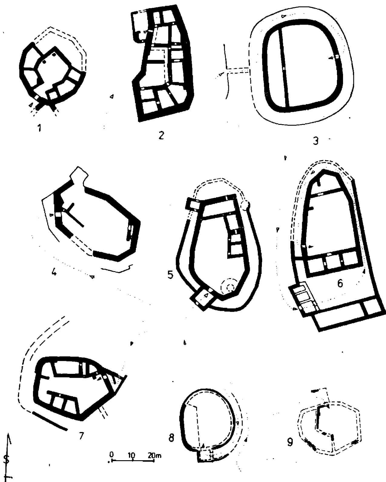
Obr. 2. Půdorysné a komunikační schéma hradů 1 - Parlčov hrad, 2 - Merkenstein (Dolní Rakousy), 3 - Gościszów (Slezsko), 4 - Divín, 5 - Helfštejn, 6 - Vikštejn, 7 - jádro hradu Gryf (Slezsko), 8 - Dalečín, 9 - Zubříž (Nový Sauburk). 2, 3, 8, 9 - podle autora, 1 - podle M. Slivky, 4 - podle L. Šáskyho, 5 - podle D. Menclové, 6 - podle O. Pipera, 7 - podle B. Guérquina.
