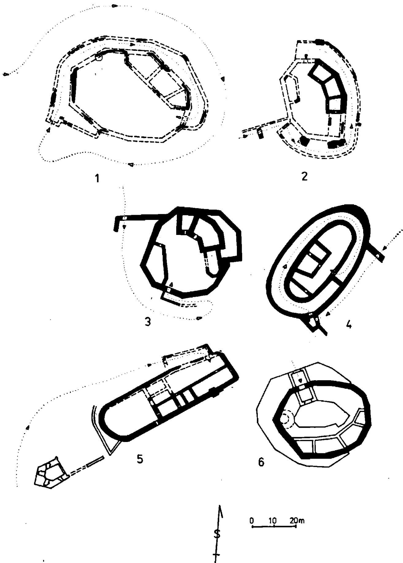
Obr. 1. Půdorysné a komunikační schéma hradů 1 – Světlov, 2 – Brničko, 3 – Oberwalsee (Horní Rakousy), 4 – Nový Hrádek n. Dyji, 5 – Děvčický, 6 – Boskovice. 1, 2, 5 – podle autora, 3 – podle G. Grüllla, 4 – výřez z plánu z archivu KSPPOP Brno, 6 – podle F. Kašíčky.
